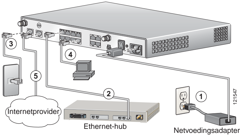
Afbeelding 2 Standaardinstallatie van een Cisco 1801-, Cisco 1802- of Cisco 1803-router
