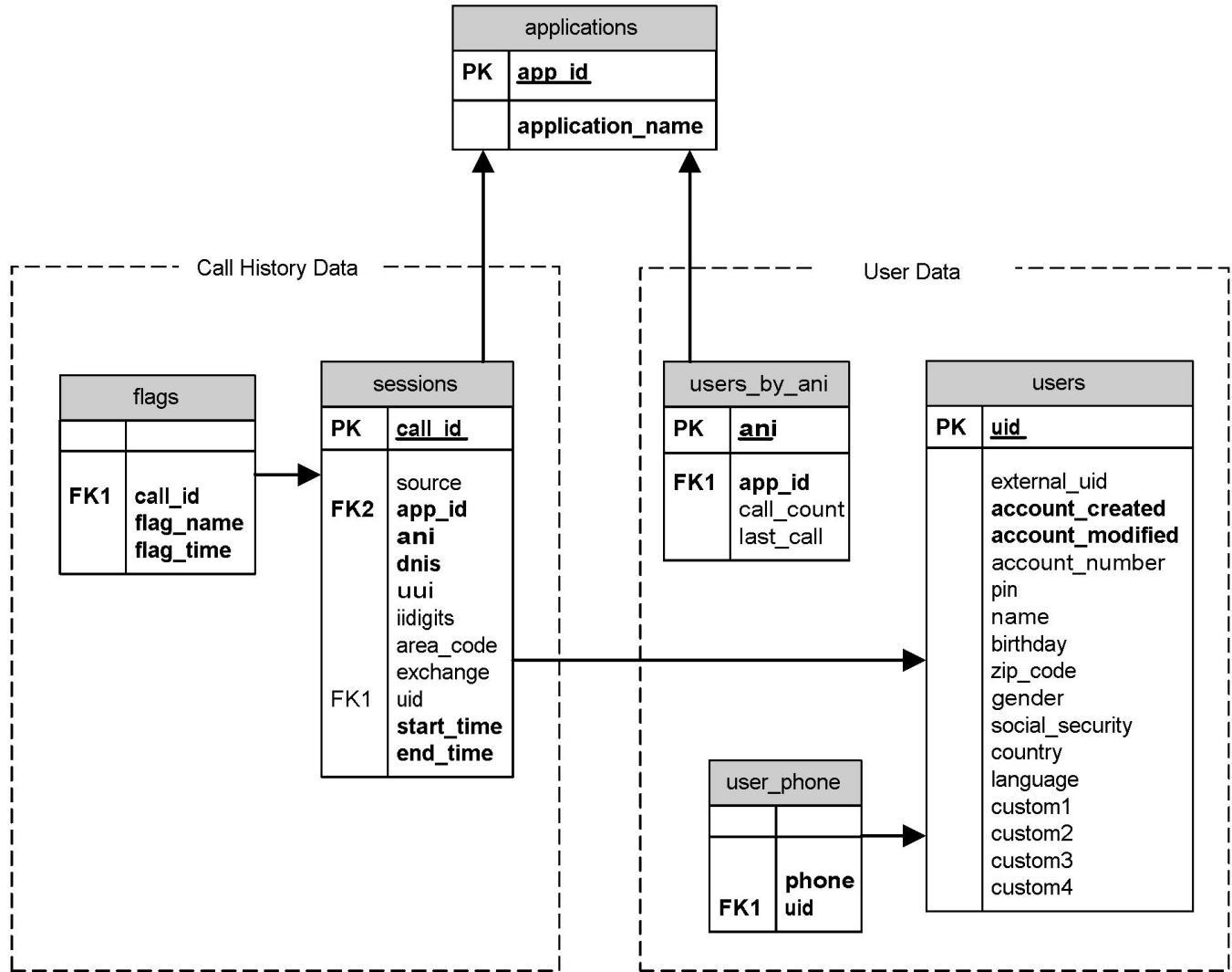
Figure 19: Database ER Diagram
