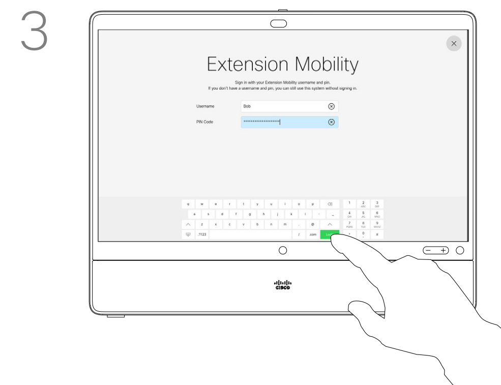
3 Tap Login .
