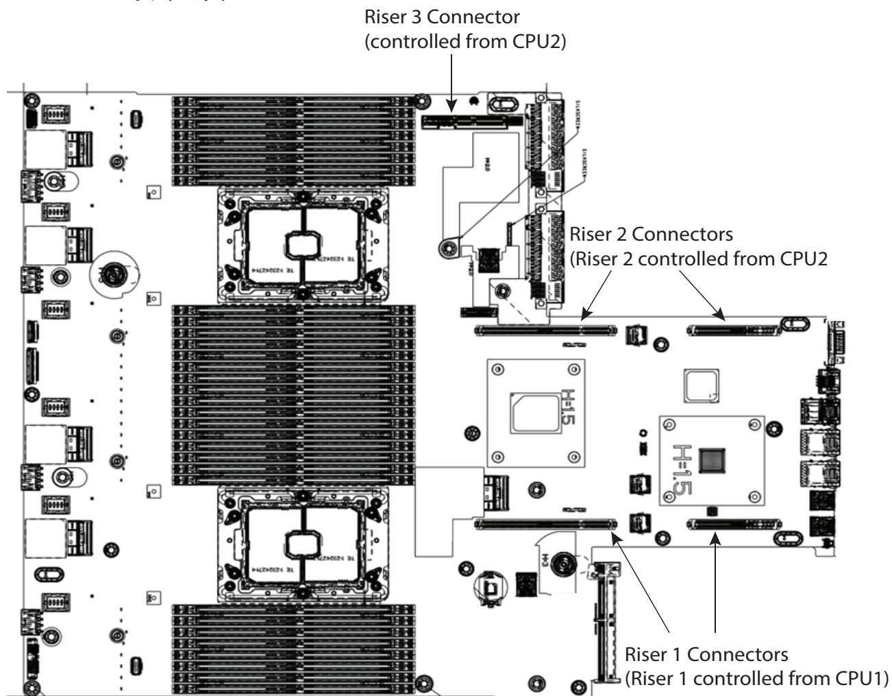
図 6 HyperFlex Express HX245C M6SX All Flash およびハイブリッド サーバー ノードのライザー コネクタの位置
