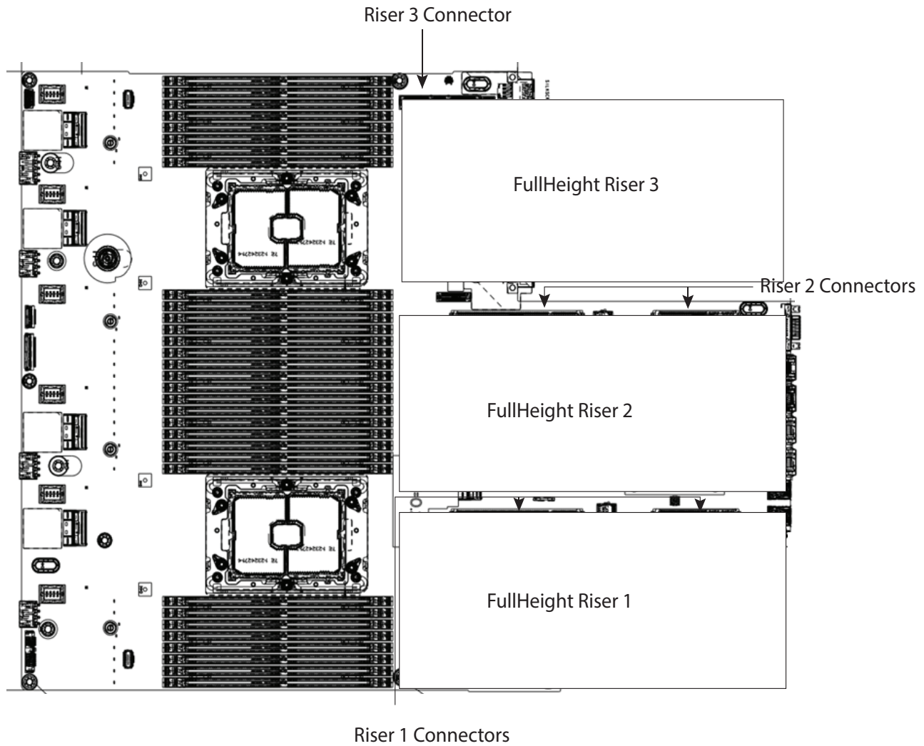
図7 3つのフルハイトライザーが接続された HyperFlex Express HX245C M6SX All Flash/ ハイブリッド サーバー ノード
