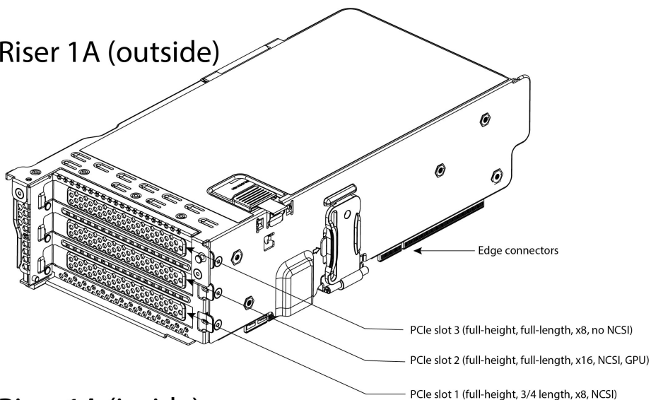
図 9 ライザー カード 1A
