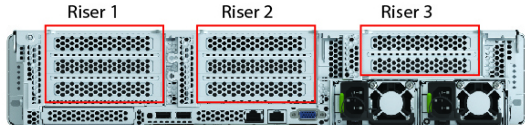
図 8 ライザー カードの場所
