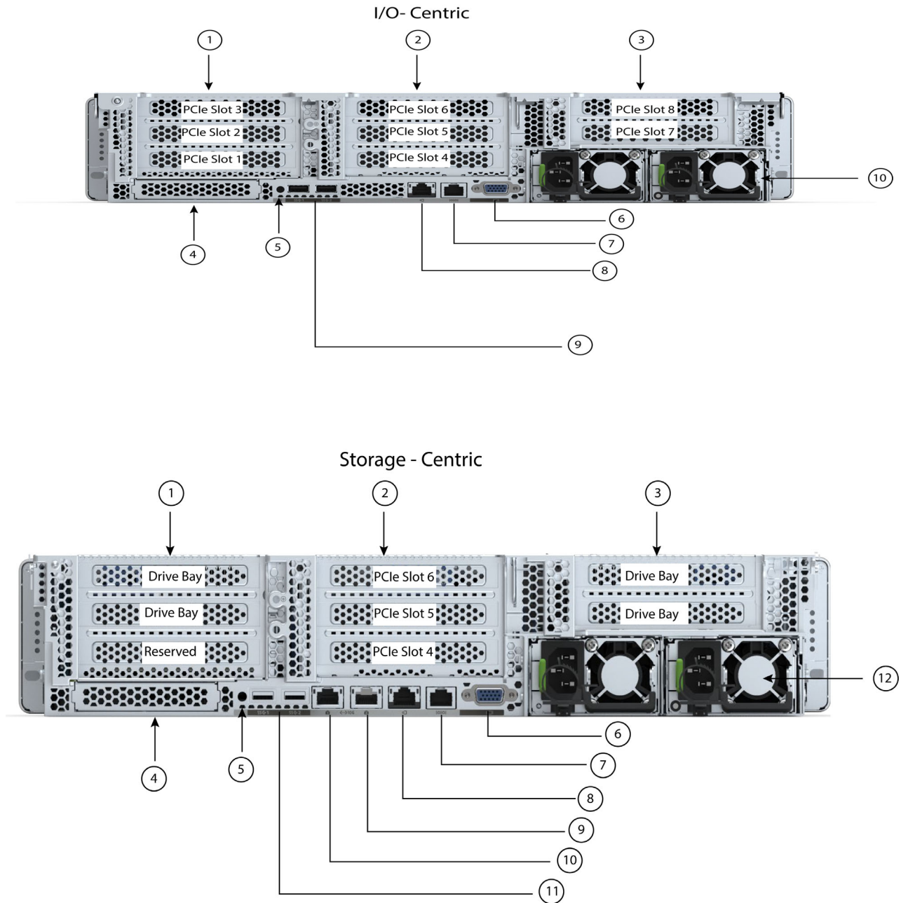
図 4 シャーシ背面図 - HX245C-M6SX-EXP (Hybrid)
