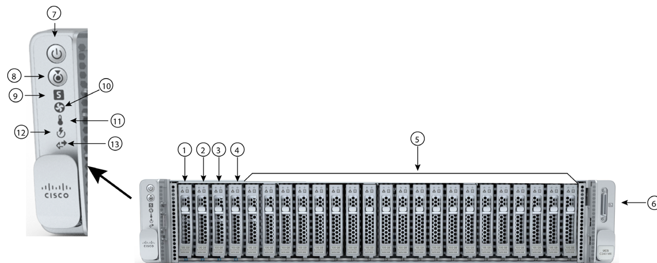
図 1 シャーシ正面図 : HXAF245C-M6SX-EXP (All Flash)
