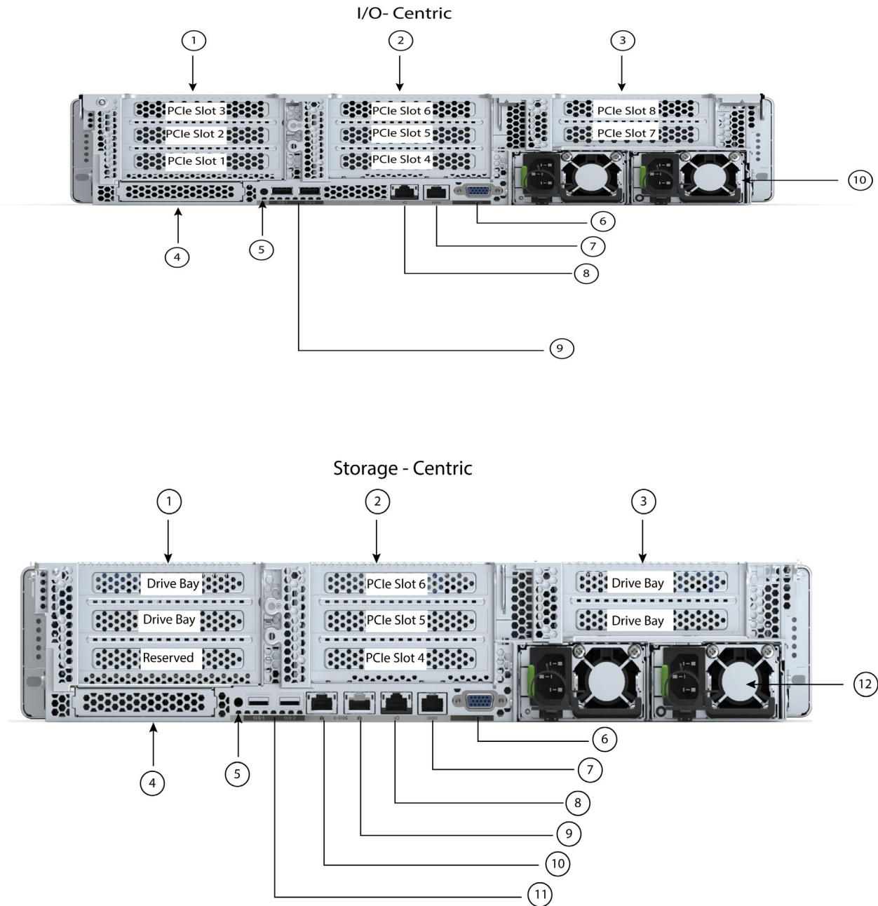
図 2 シャーシ背面図 : HXAF245C-M6SX-EXP (All Flash)
