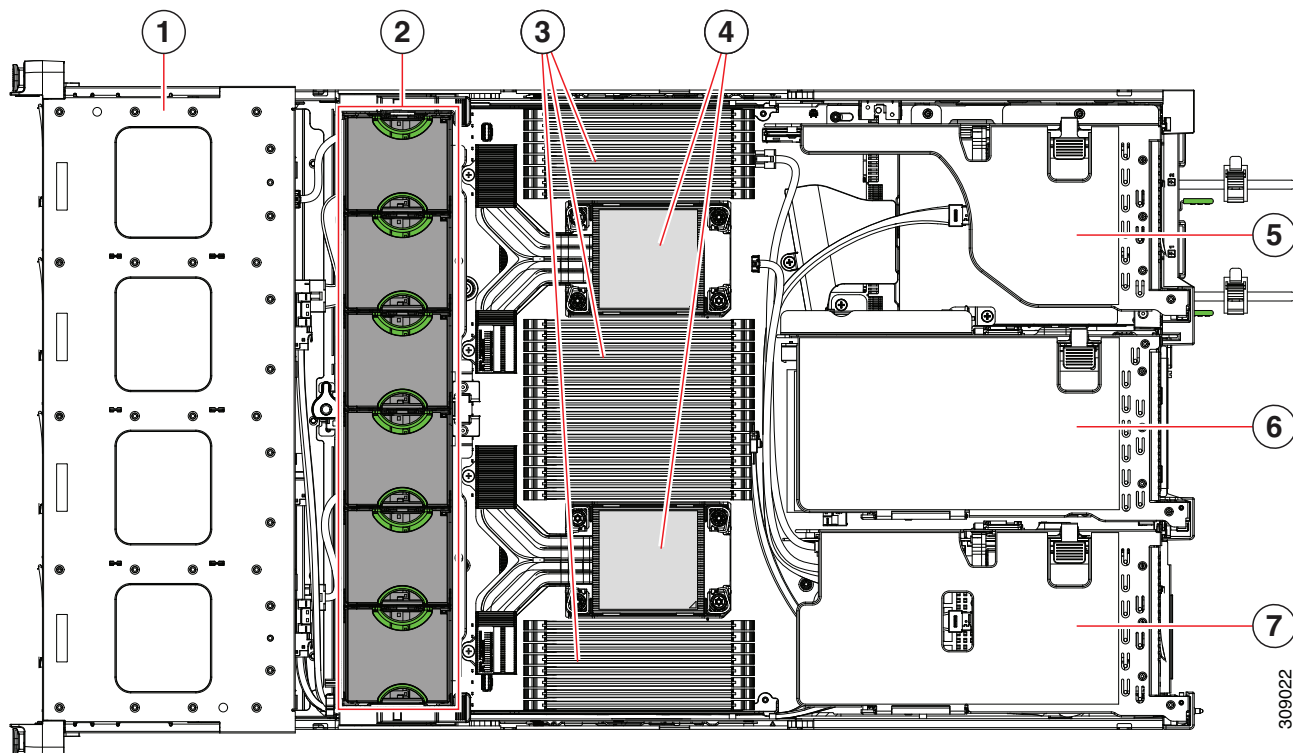
図 5 トップカバーがオフの Cisco HyperFlex HX245C M6SX All Flash およびハイブリッド サーバーノード
