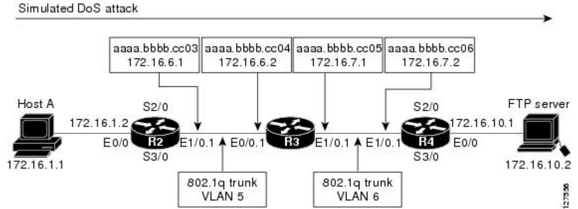
Figure 2 Simulated DoS Attack (d)
