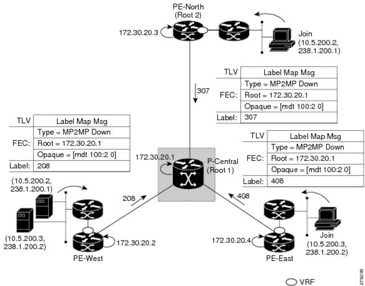
Figure 35: Default MDT Downstream--Root 1
