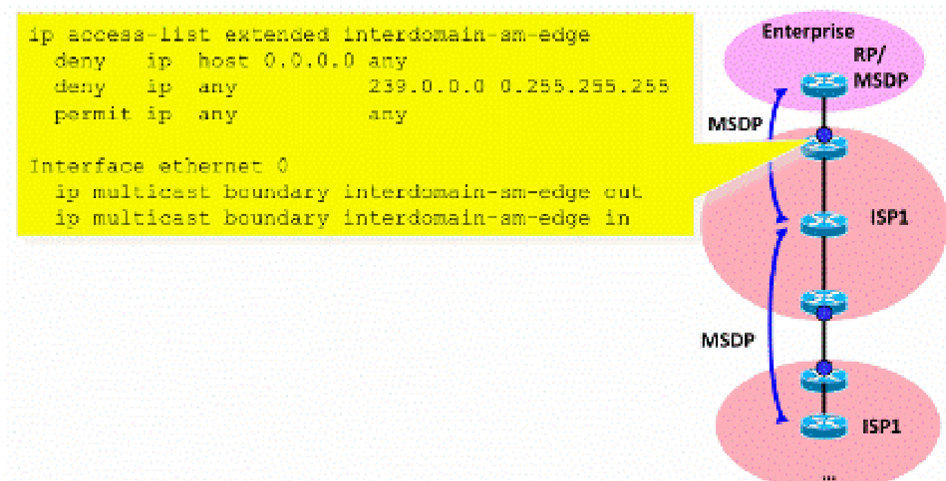
Figura 13: Filtro entre dominios (*,G)
