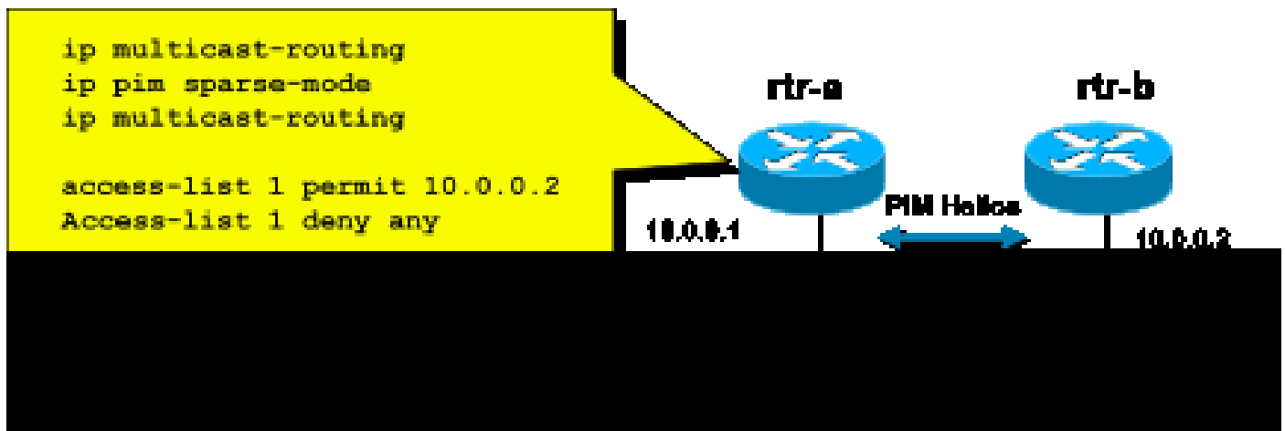
Fig. 7: Control de vecino PIM
