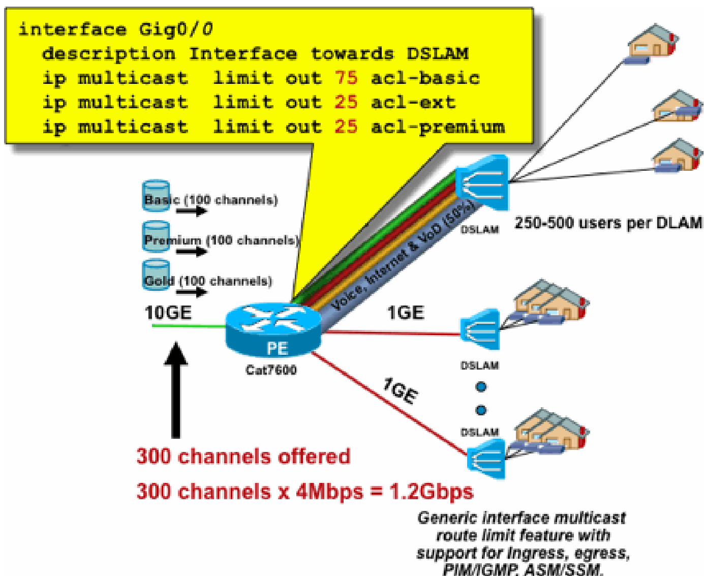
Fig. 21: Uso de límites de ruta multicast por interfaz; Control de admisión en link Agg-DSLAM
