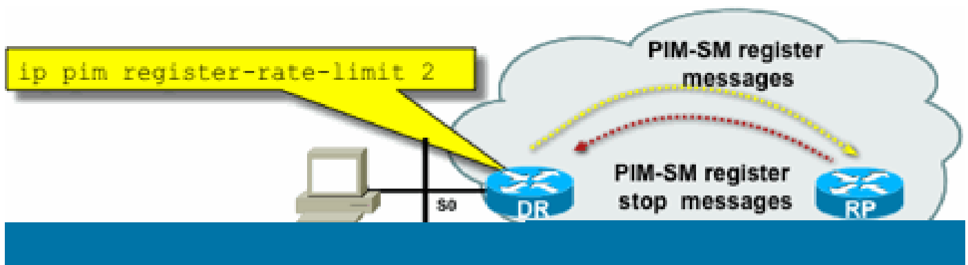
Fig. 8: Control del túnel de registro PIM-SM
