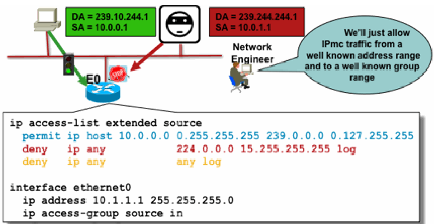
Figura 16: Fuentes de control
