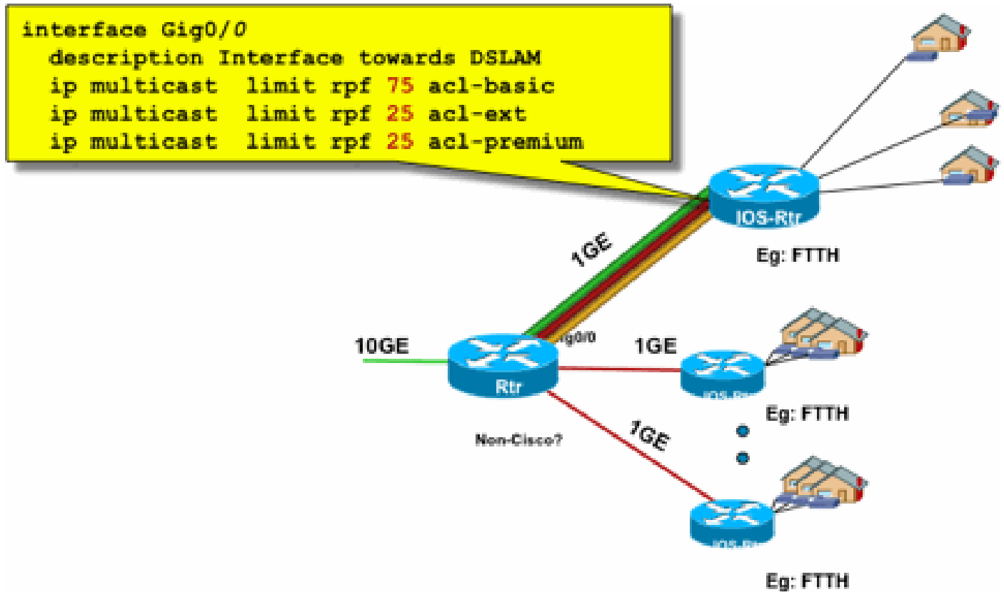
Fig. 22: Uso de límites de ruta multicast por interfaz; Control de admisión de entrada
