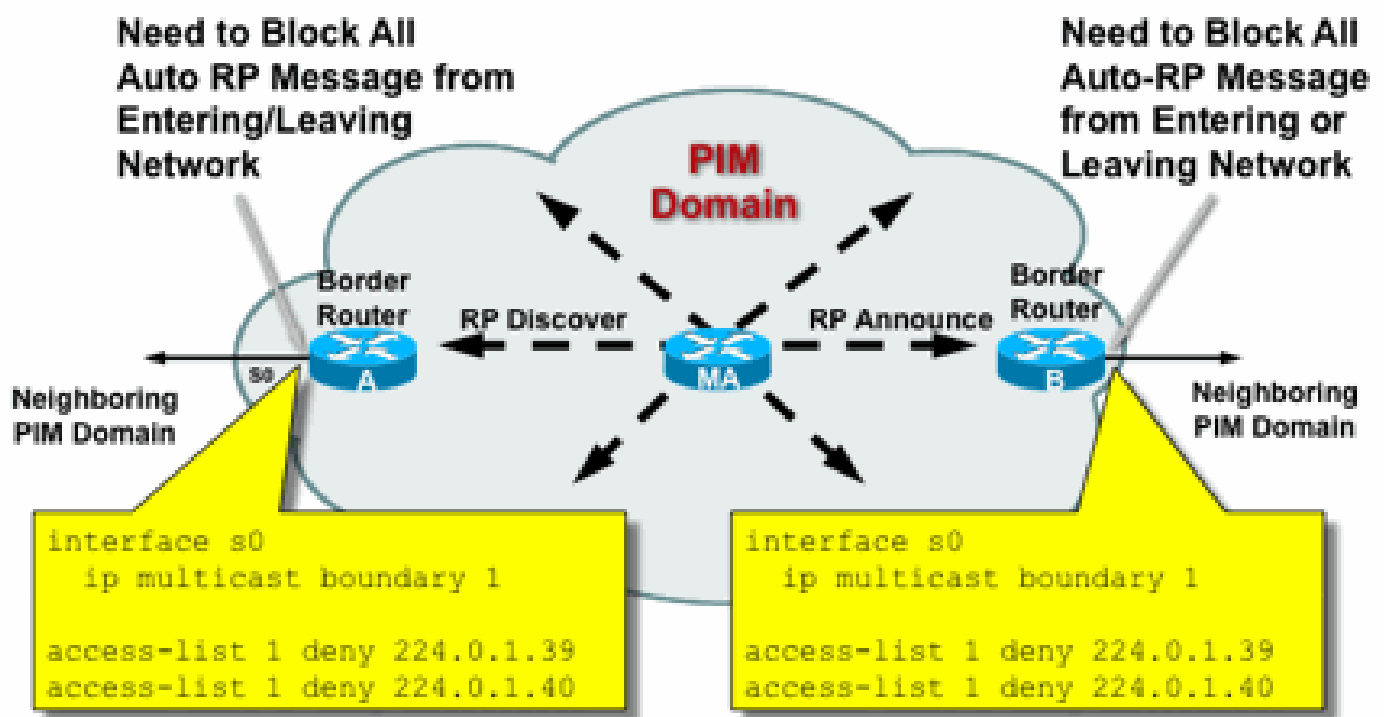
Figura 10: Comando de límite de multidifusión
