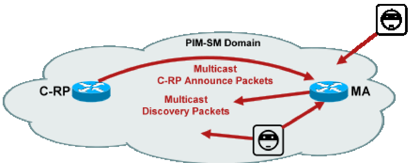
Figura 2: Paquetes RP automáticos
