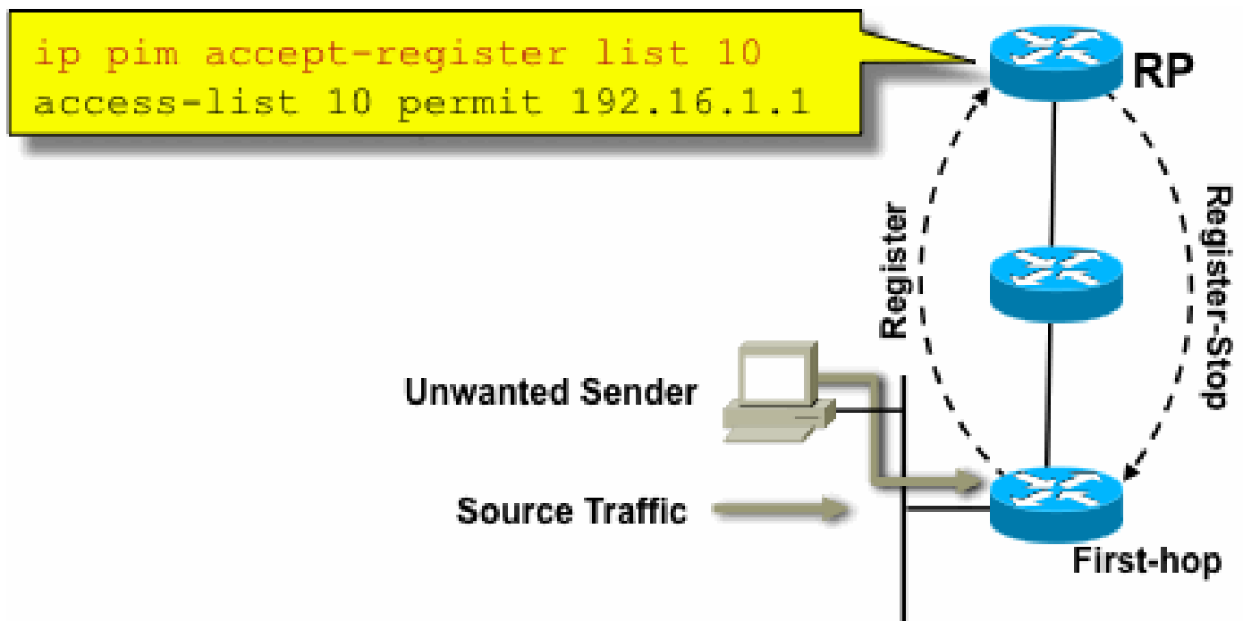
Fig. 17: Control de fuente PIM-SM
