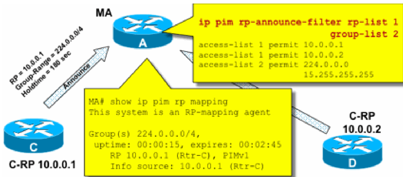
Fig. 9: Auto-RP - Filtro de anuncio RP
