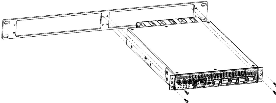
Illustration 9 : Fixation de l'assemblage
