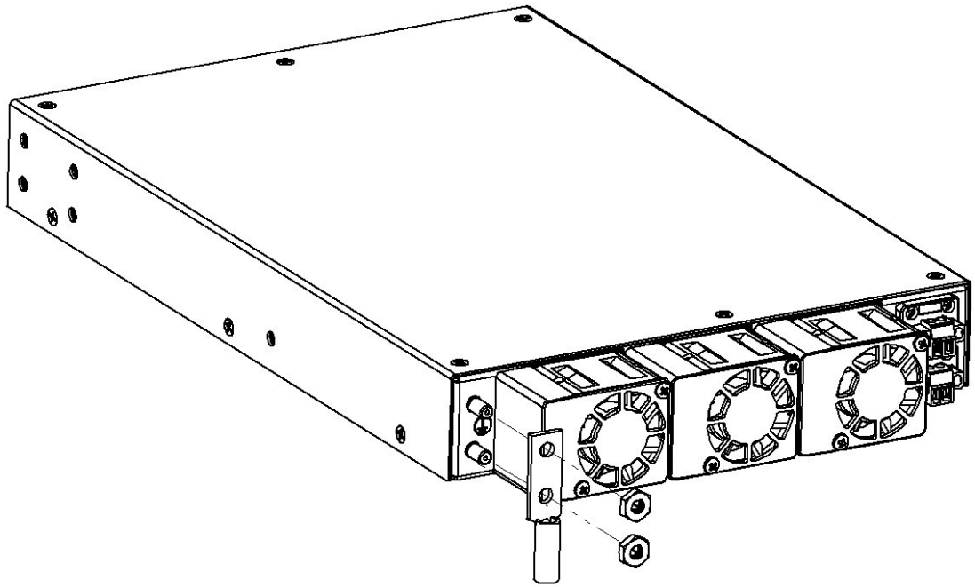
Illustration 10 : Fixation de la cosse de mise à la terre
