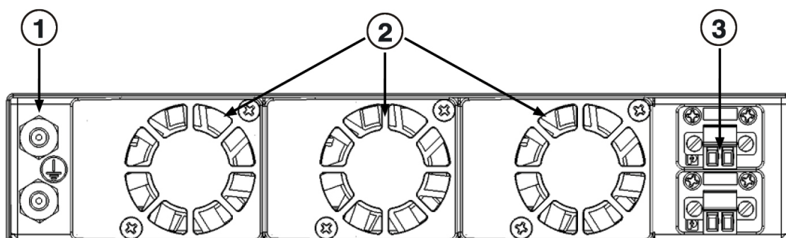
Illustration 5 : Alimentation CC
