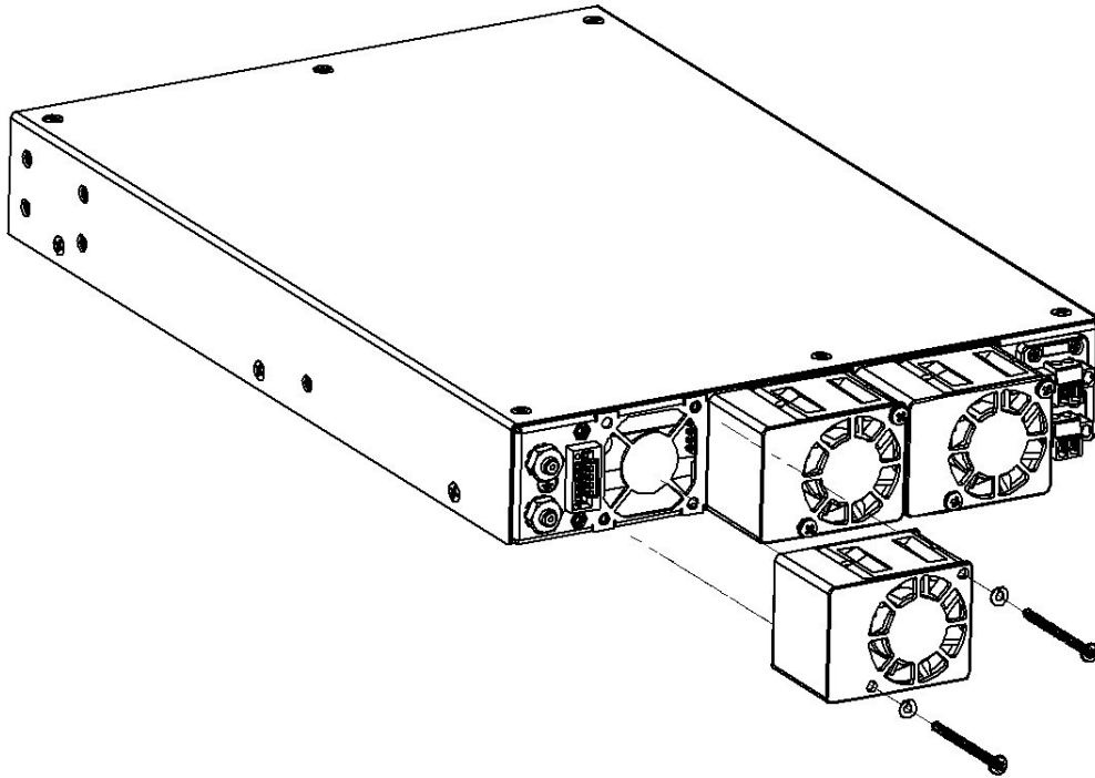
Illustration 11 : Retrait du ventilateur
