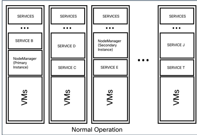
Figure 28: Scénario de défaillance d'un service
