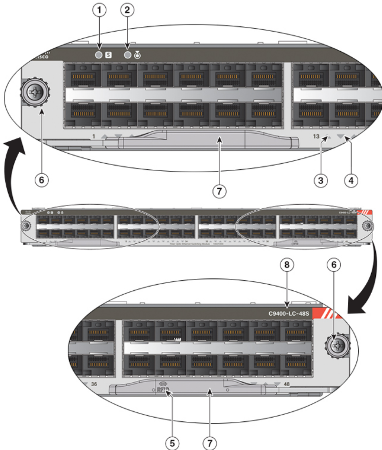
Illustration 15 : Vue de face de la carte de ligne C9400-LC-48S
