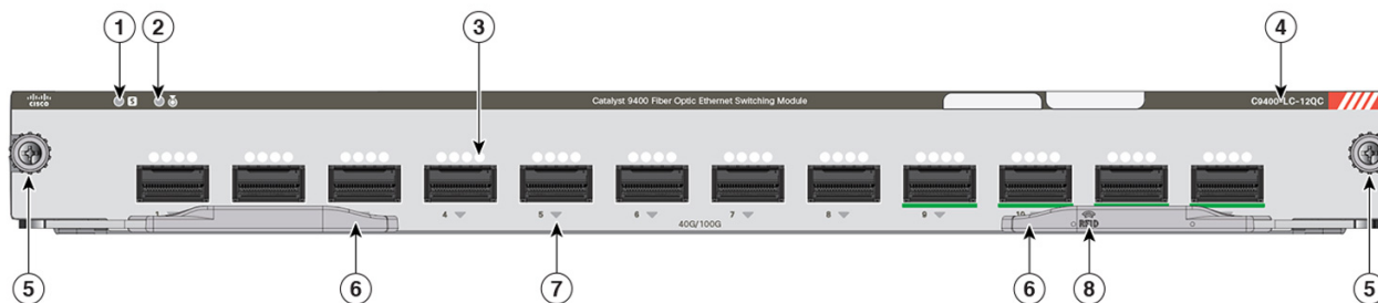
Illustration 9 : Vue de face de la carte de ligne C9400-LC-12QC
