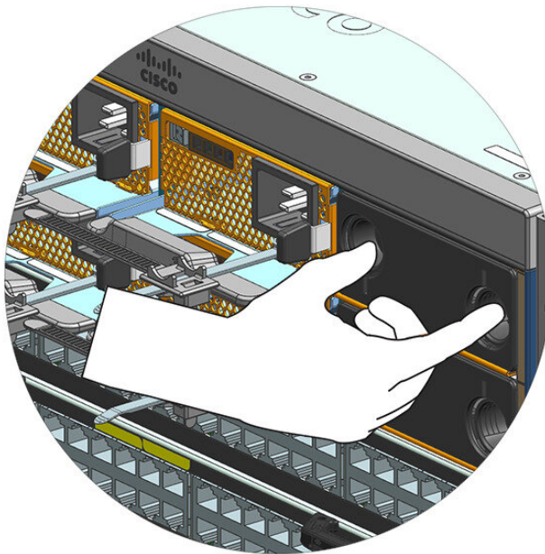
Illustration 35 : Retirer un cache d'alimentation
