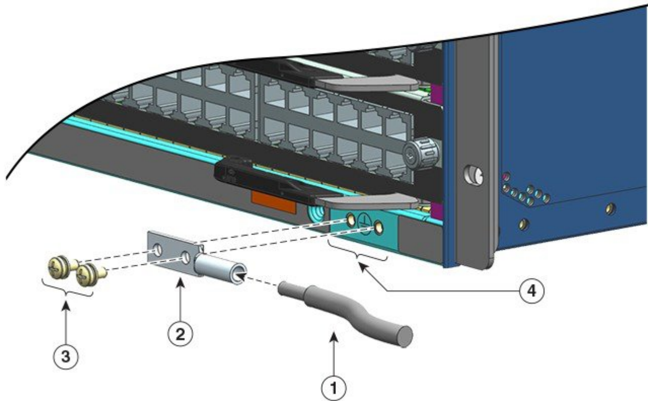
Illustration 28 : Identifier et connecter le système de mise à la terre
