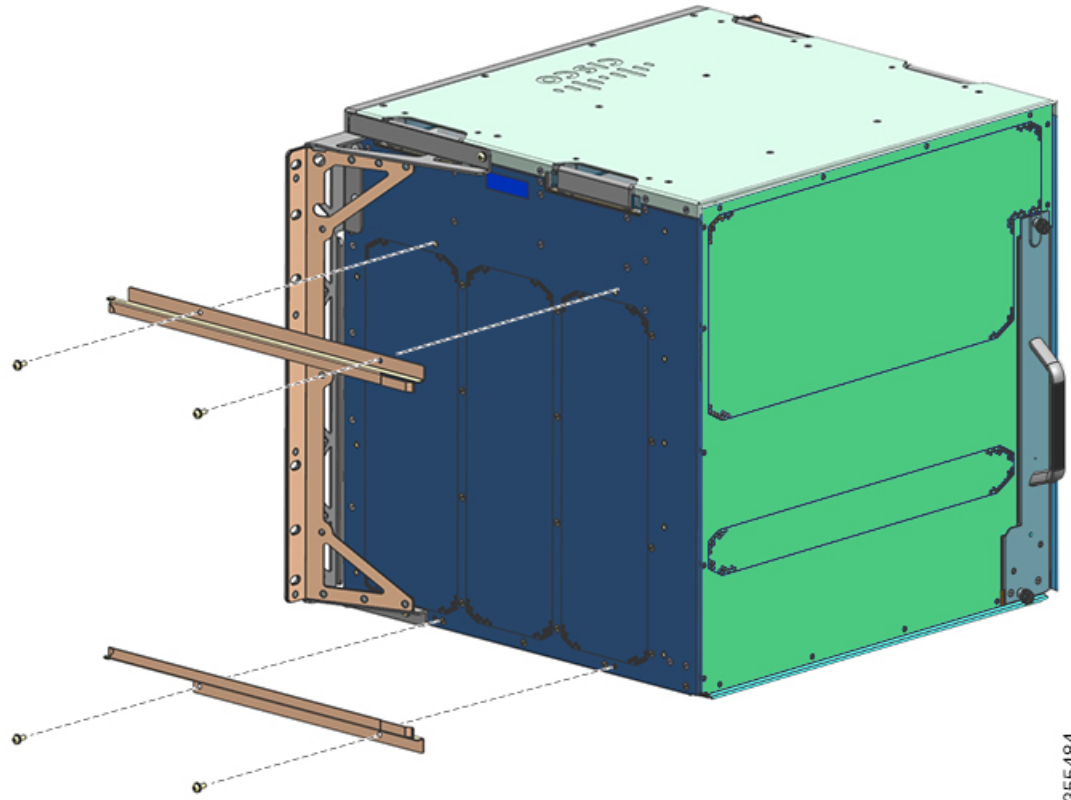
Illustration 23 : Installer les supports de filtre
