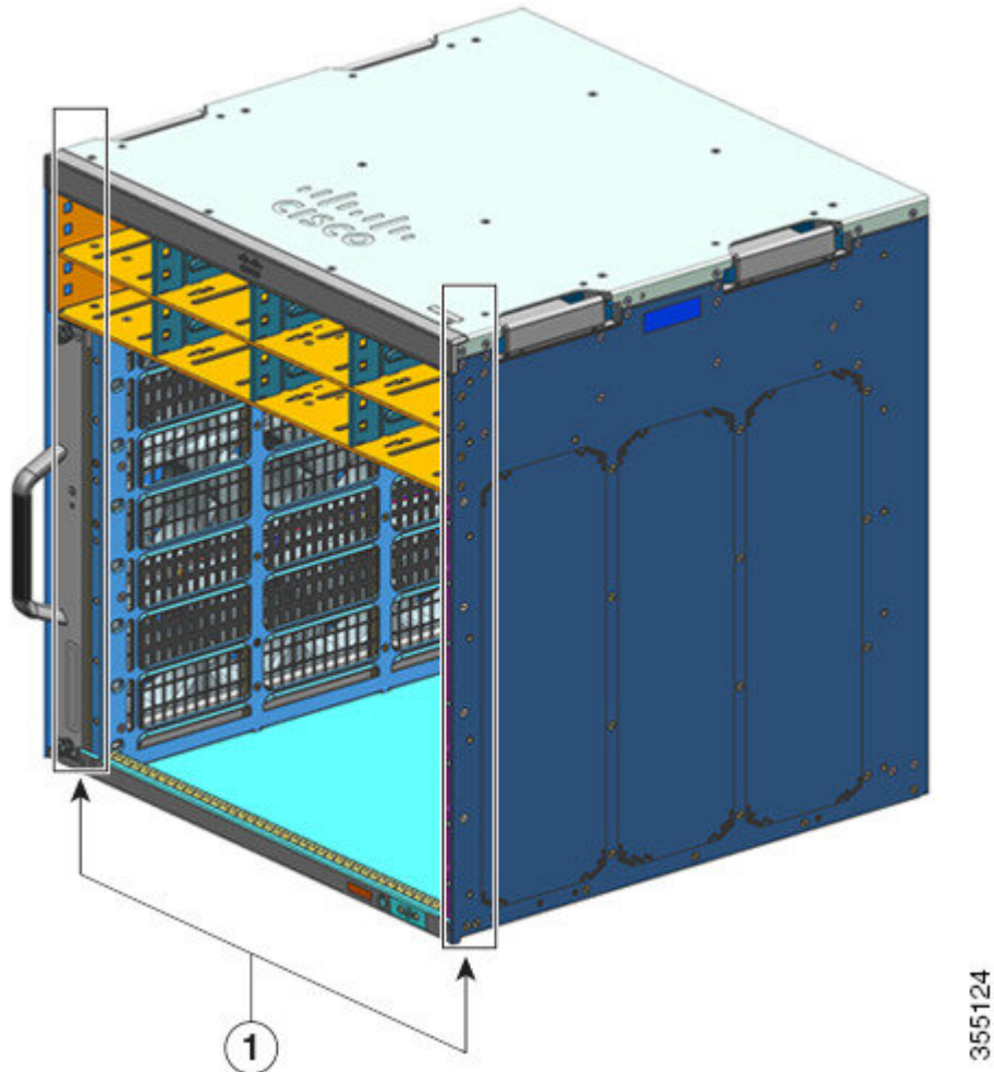
Illustration 13 : Châssis sans les supports en L
