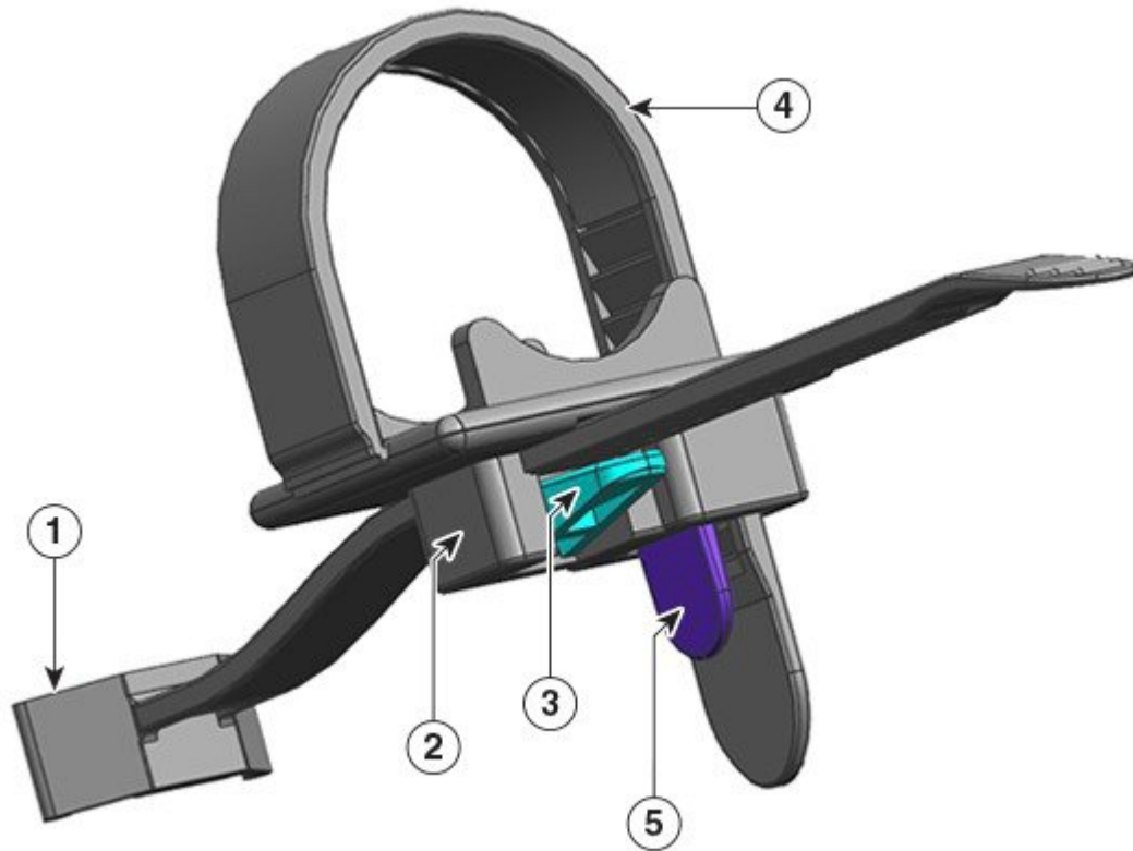
Illustration 30 : Composants du mécanisme de maintien du câble d'alimentation
