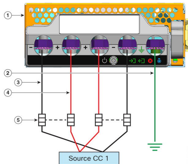
Illustration 7 : Exemple d'installation C9400-PWR-3200DC – Source d'alimentation CC unique
