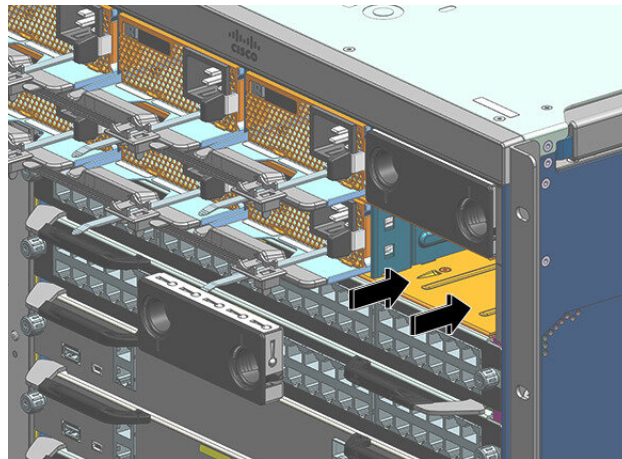
Illustration 37 : Cache d'alimentation installé
