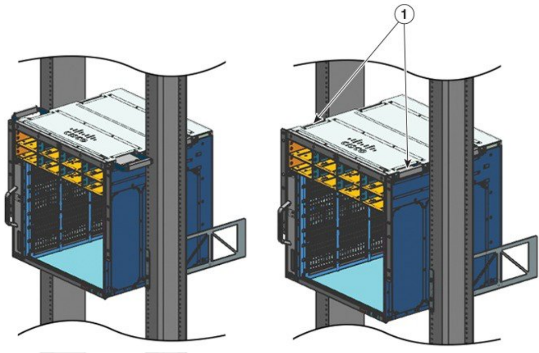
Illustration 18 : Insérer le châssis – Partie 2
