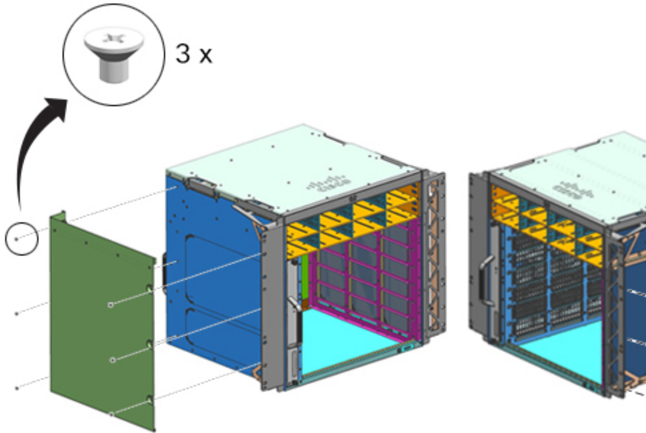
Illustration 24 : Installer les panneaux de protection
