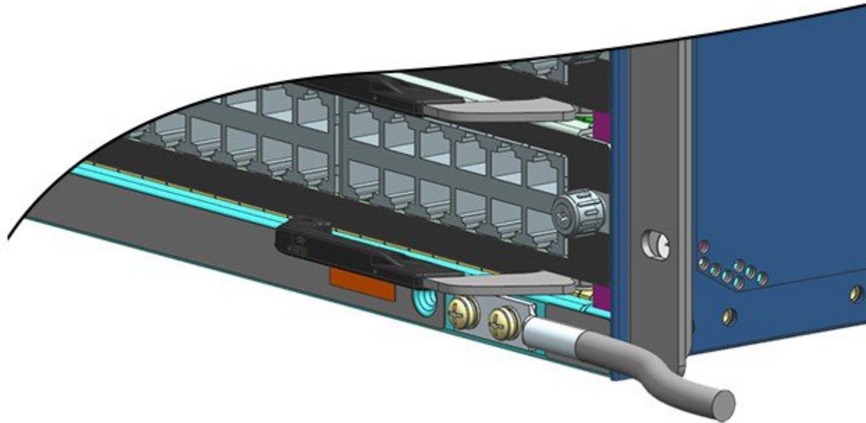
Illustration 29 : Point de terre du système connecté
