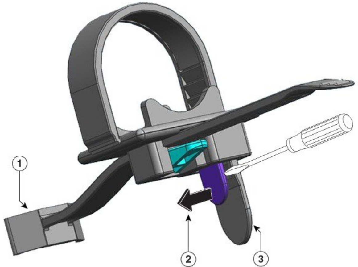
Illustration 33 : Bride de maintien flexible
