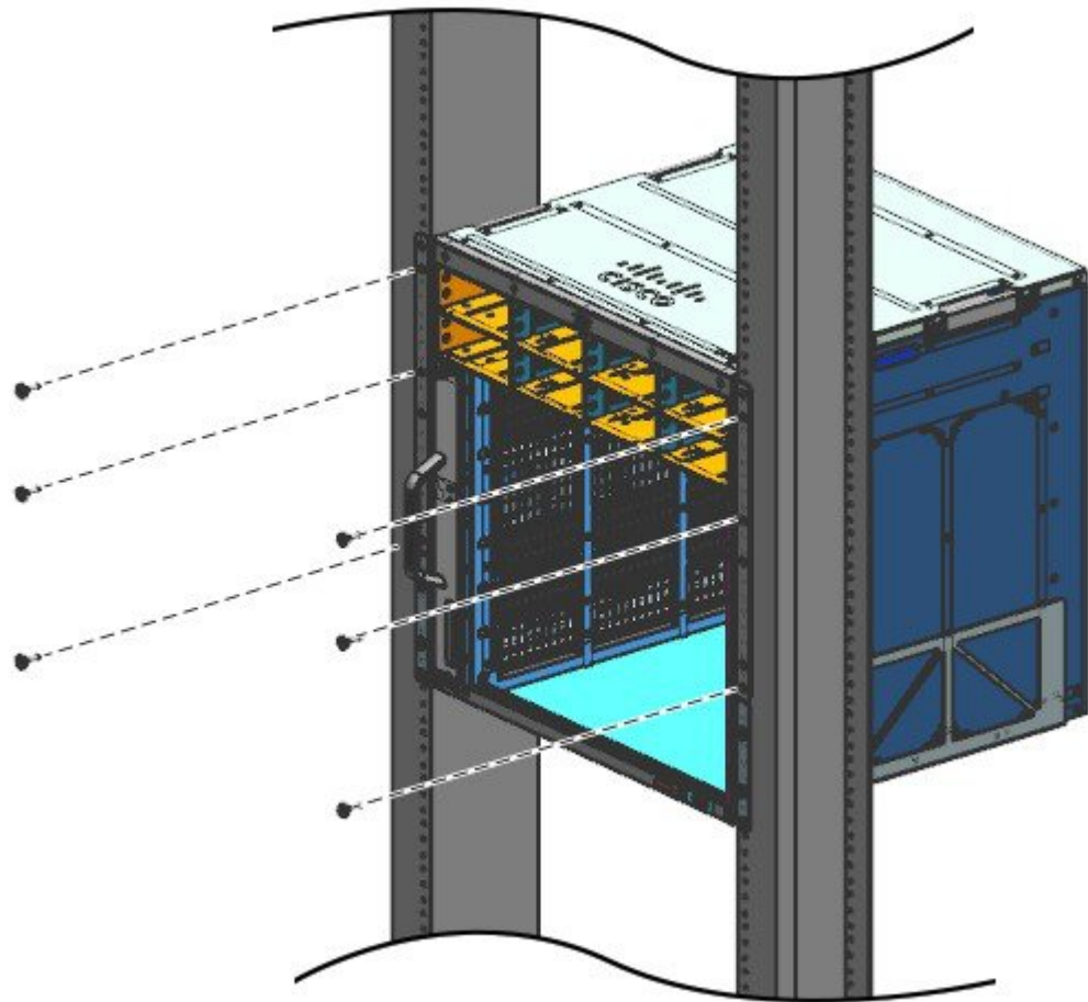
Illustration 19 : Fixer le châssis aux montants du rack
