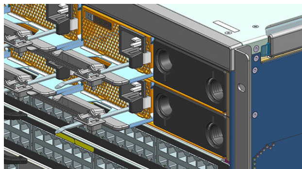
Illustration 37 : Cache d'alimentation installé
