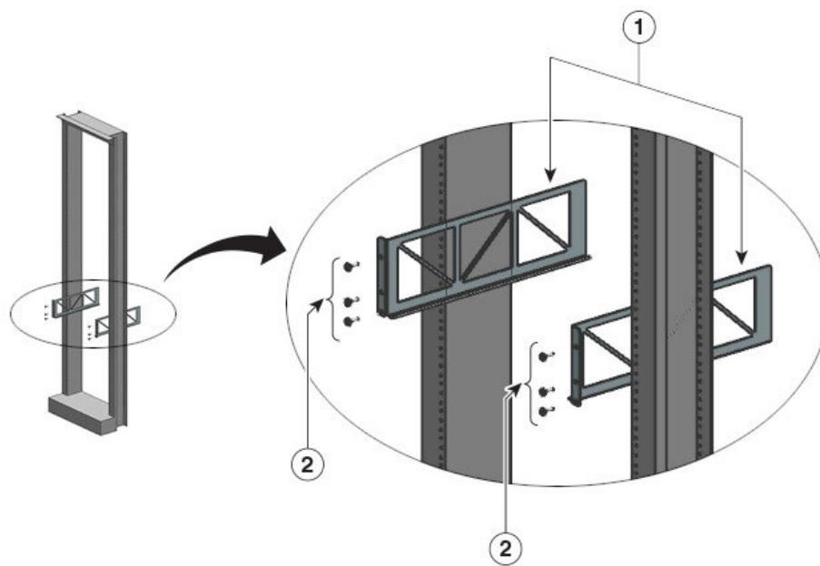
Illustration 15 : Installer les supports de tablette
