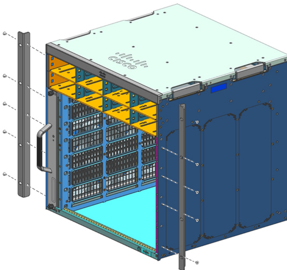
Illustration 21 : Retirer les étriers
