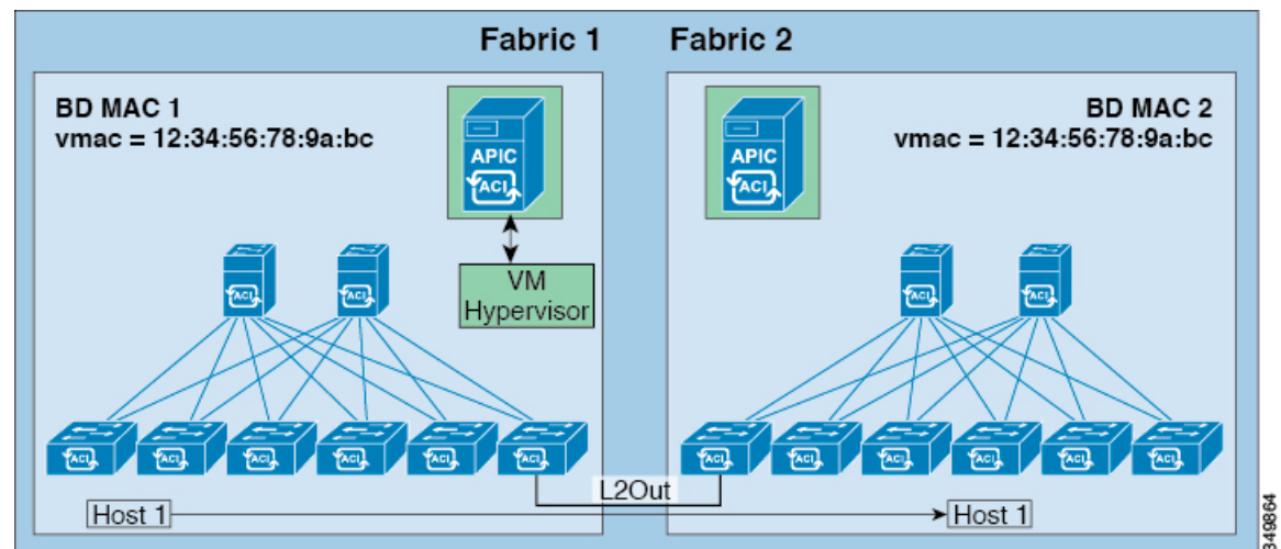
図 8: ACI マルチファブリック共通パーベシブゲートウェイ
