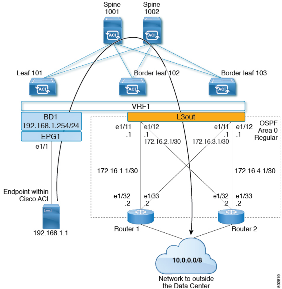
図 2: 2つの外部ルータがある OSPF L3out のトポロジ例
