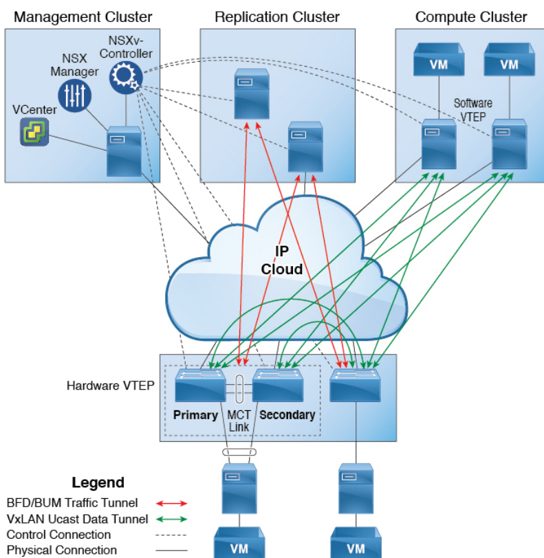
図 9: VLAN トンネルモードの Cisco ACI の課題
