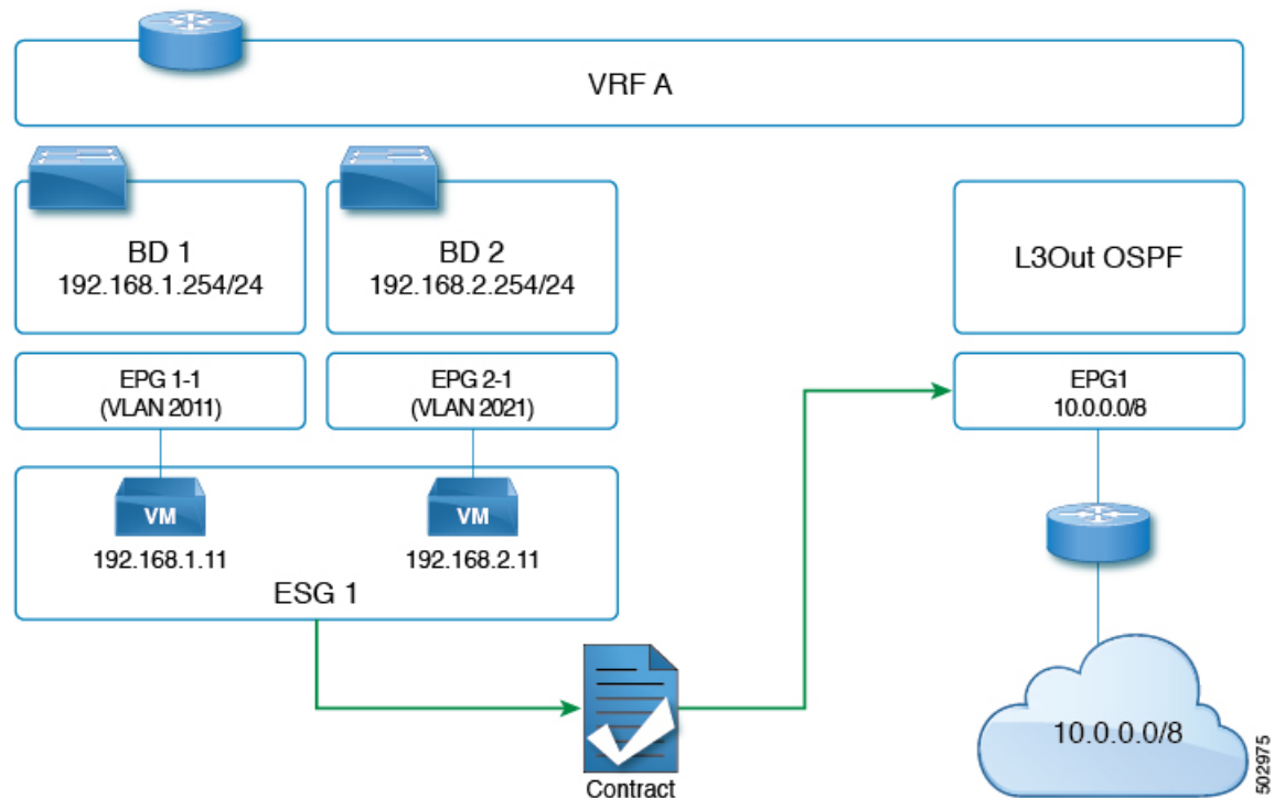
図 8: ESG から外部への接続は、L3 外部 EPG を使用して実装されます。
