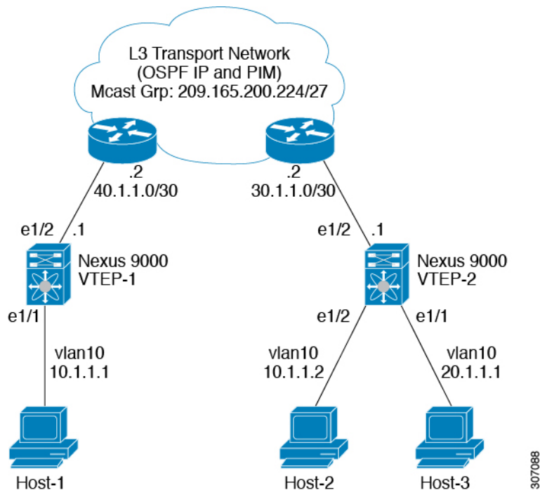
図 5: VXLAN Decap スイッチのレイヤ3 VNI の VLAN ACL
