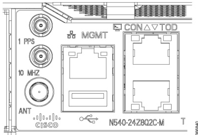
図 1 : Cisco NCS 540 シリーズ ルータ前面パネルの 1PPS、10MHz、および ToD ポート
