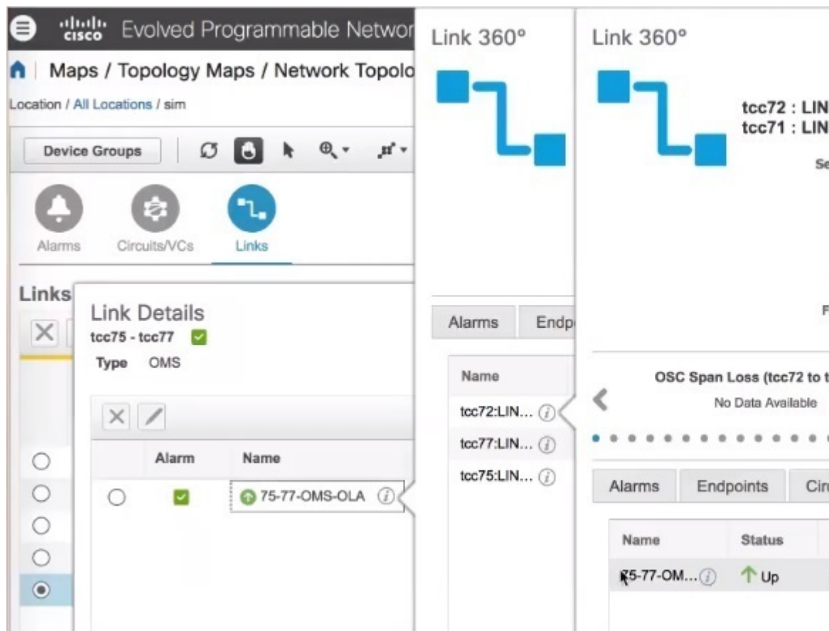
図 3: [リンクの詳細 (Link Details)] と [リンク 360* (Link 360*)] ビュー
