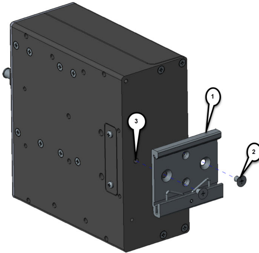
図 11: 垂直に取り付ける場合の DIN レールブラケットの取り付け
