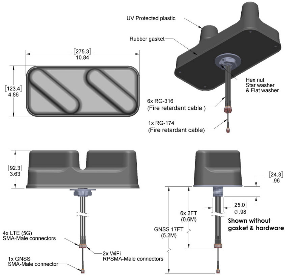
図 2: Cisco ANT-7-5G4WL2G1-0 の機械的詳細
