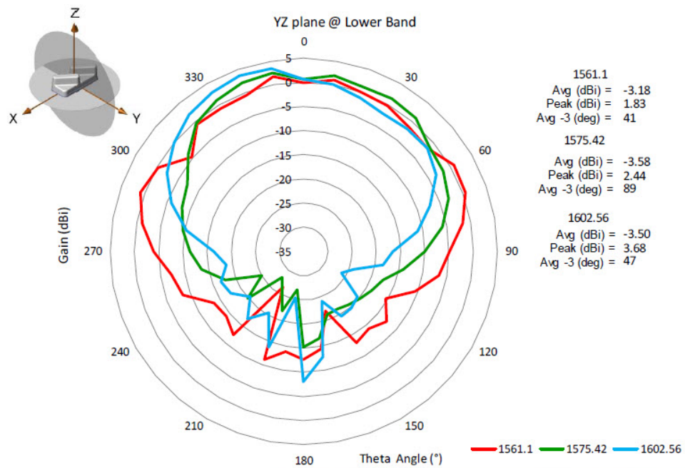
図 31 : YZ 平面 @ 低帯域
