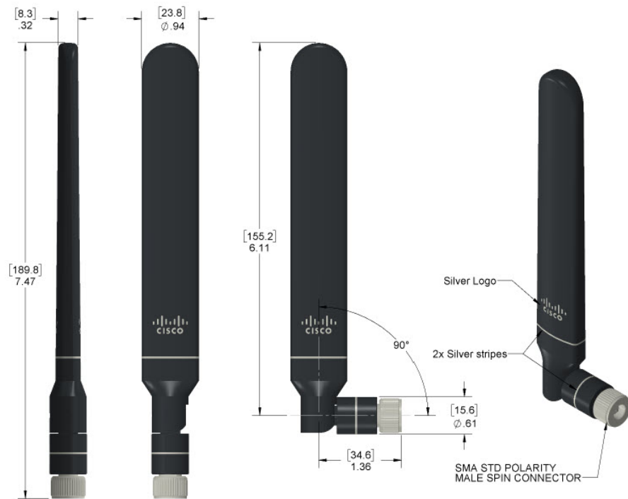
図 2: 機械図面
