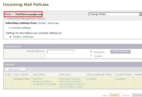
図 2: GUIの中央集中型管理機能：設定が規定されていない場合
