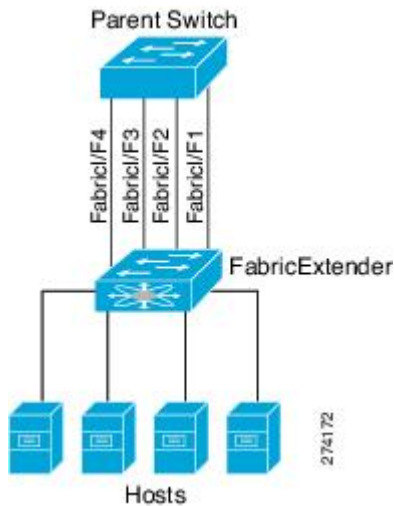
図 4： 静的ピン接続ファブリック インターフェイス接続
