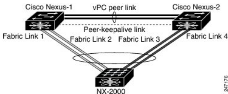
図 2: デュアルホーム接続 ファブリック エクステンダ vPC トポロジ
