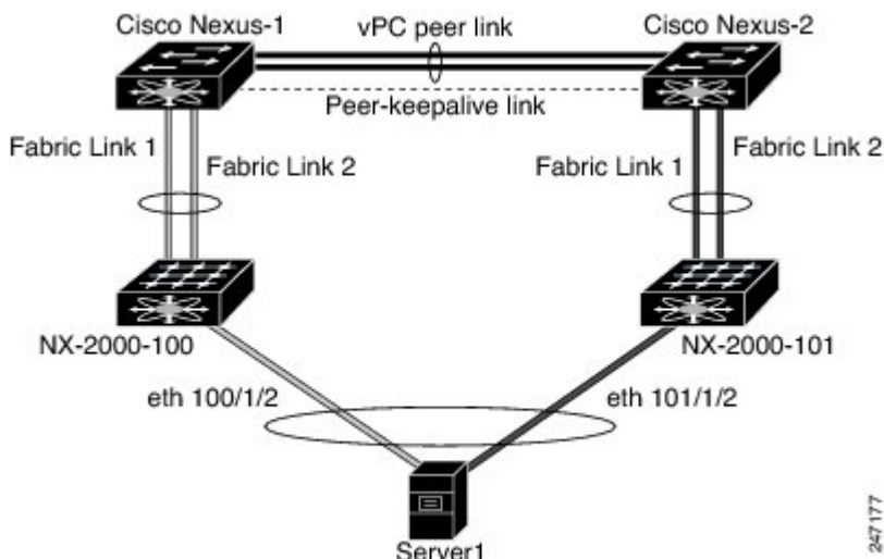
図 1: シングルホーム接続 ファブリック エクステンダ vPC トポロジ
