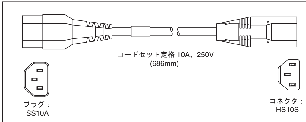
図 C-15 CAB-C13-C14-JMPR、ジャンパ電源コード
