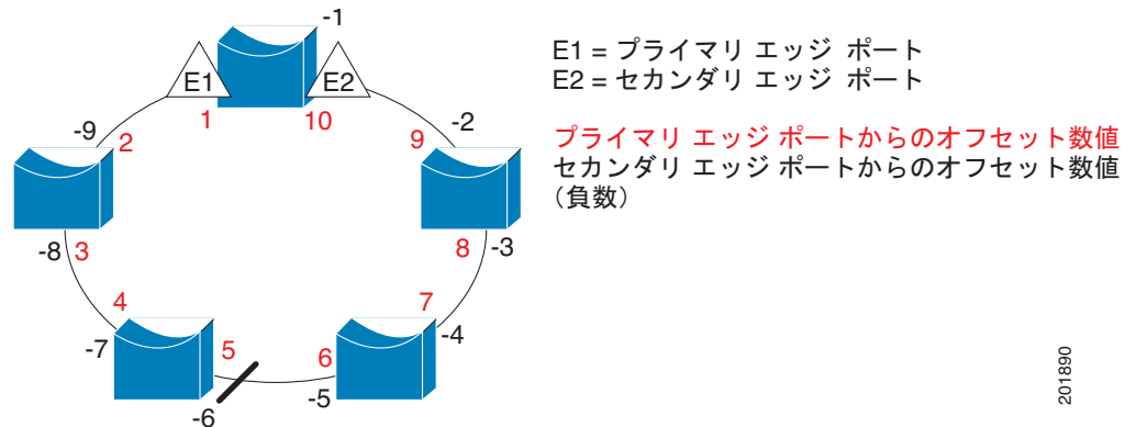
図 22-4 セグメント内のネイバー オフセット番号
