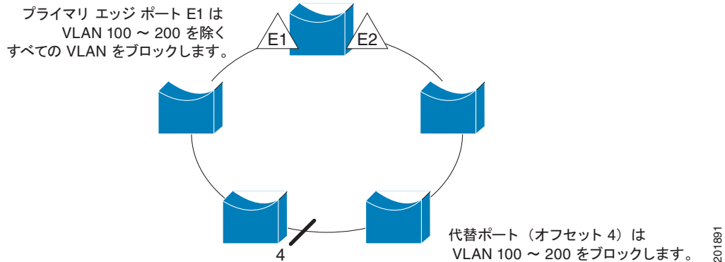
図 22-5 VLAN ブロッキングの例
