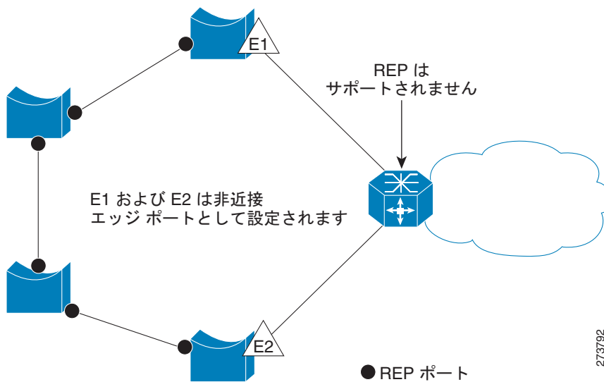
図 22-3 非ネイバー エッジ ポート
