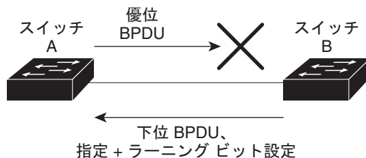
図 16-3 単一方向リンクの失敗の検出
