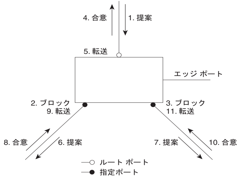
図 16-5 高速コンバージェンス中の一連のイベント
