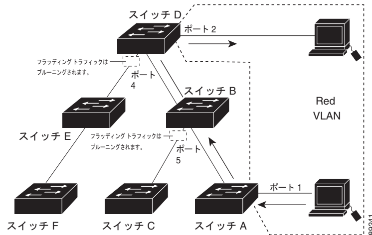
図 14-2 VTP プルーニングによるフラッディング Traffic の最適化
