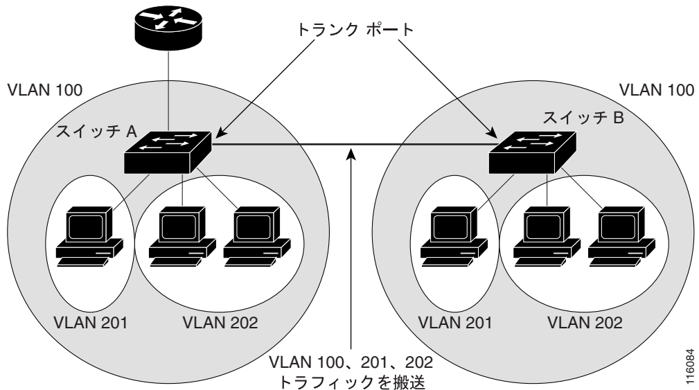
図 15-2 複数のスイッチにまたがるプライベート VLAN
