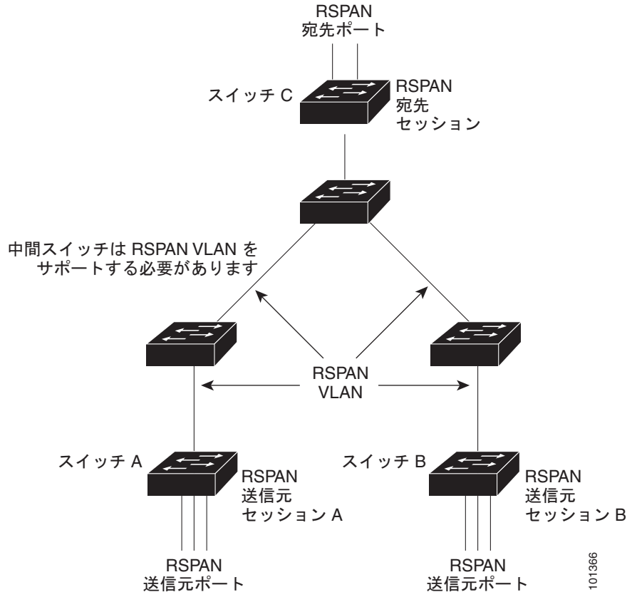
図 29-2 RSPAN の設定例
