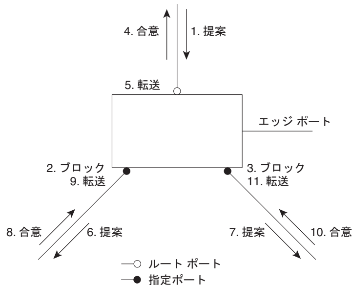
図 18-5 高速コンバージェンス中のイベントのシーケンス
