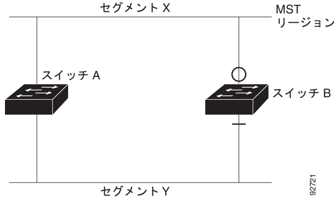
図 18-2 標準スイッチおよび先行標準のスイッチでの相互運用
