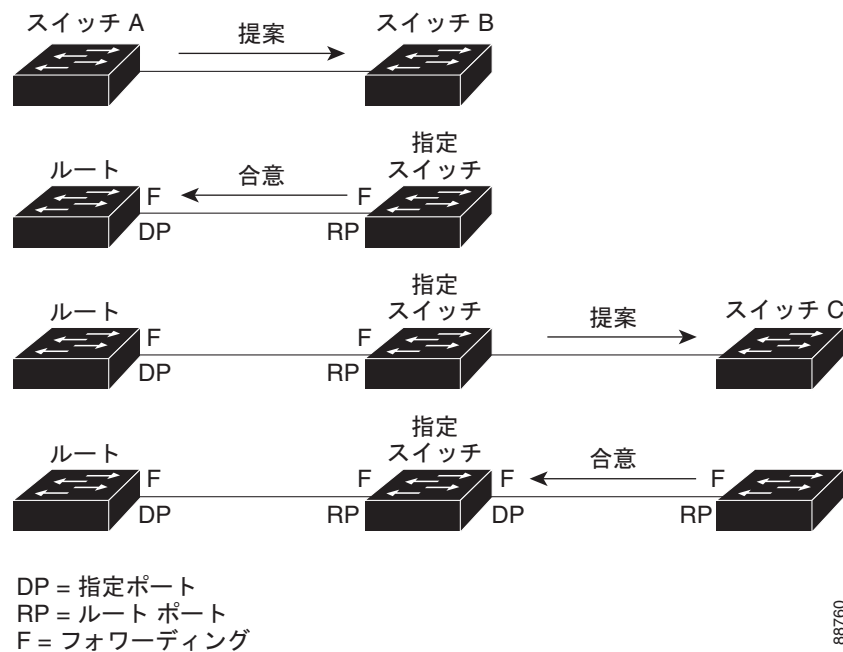
図 18-4 高速コンバージェンスの提案と合意のハンドシェイク
