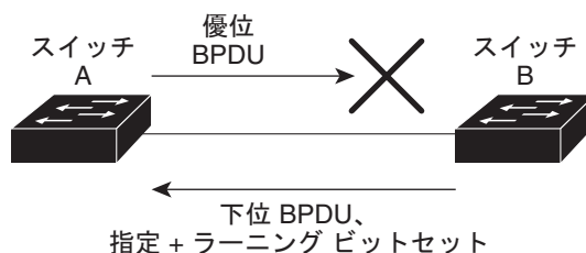
図 18-3 単一方向リンク障害の検出
