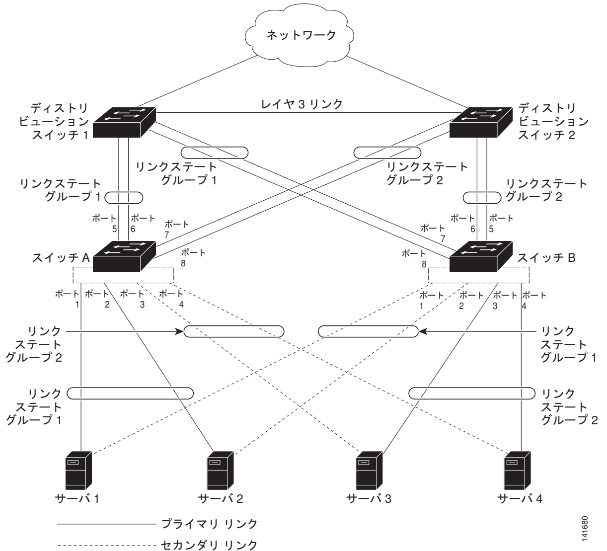
図 34-4 一般的なリンクステートトラッキングの設定
