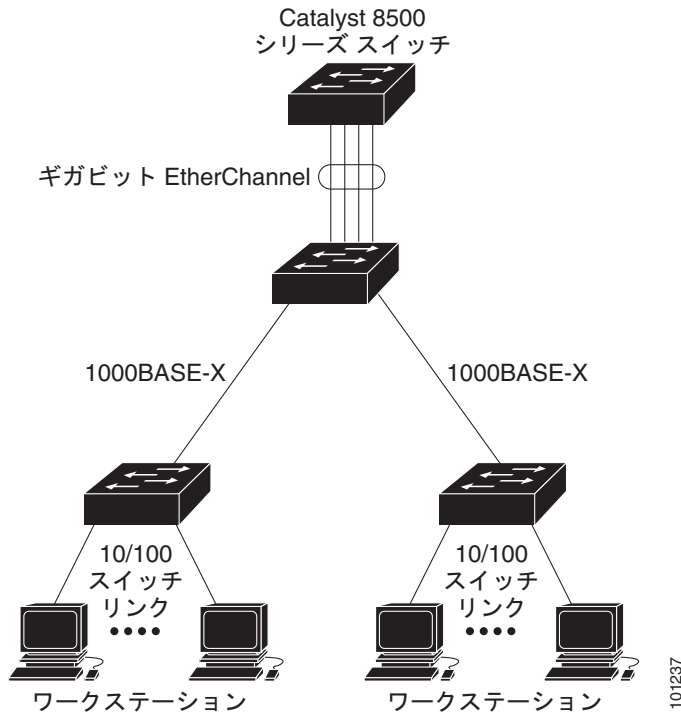
図 34-1 一般的な EtherChannel 構成
