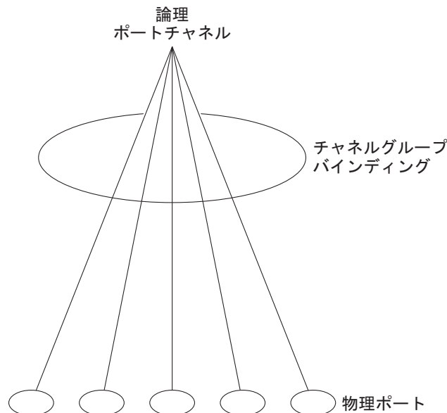
図 34-2 物理ポート、論理ポートチャネル、およびチャネル グループの関係
