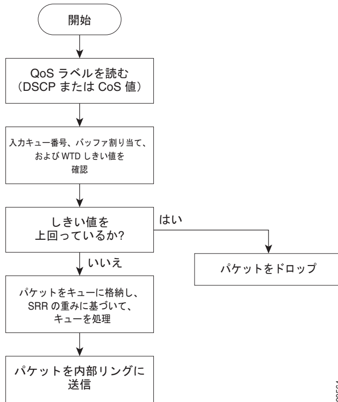
図 33-8 入力ポートのキューイングおよびスケジューリング フローチャート
