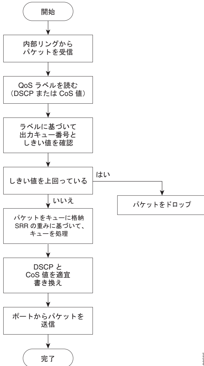
図 33-9 出力ポートのキューイングおよびスケジューリング フローチャート
