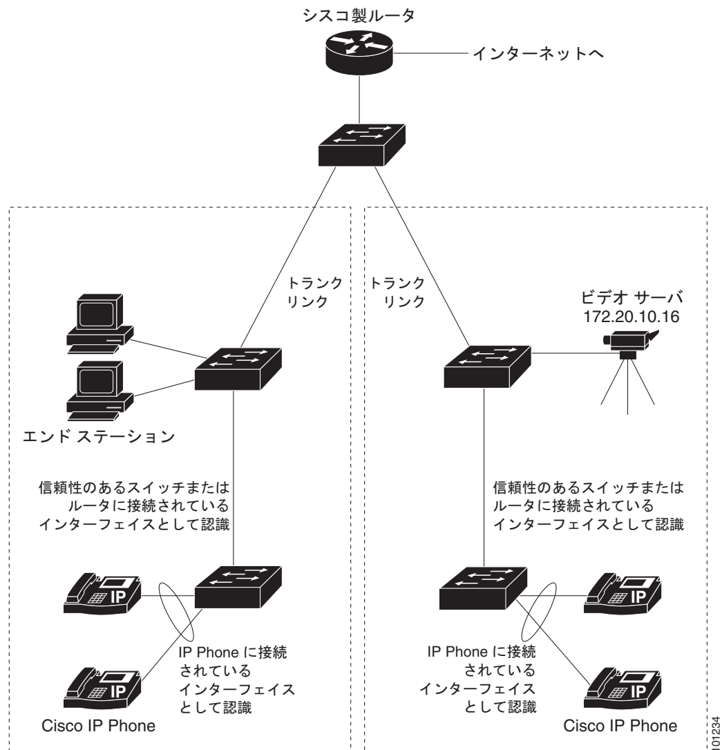
図 33-11 ネットワークでの自動 QoS の設定例
