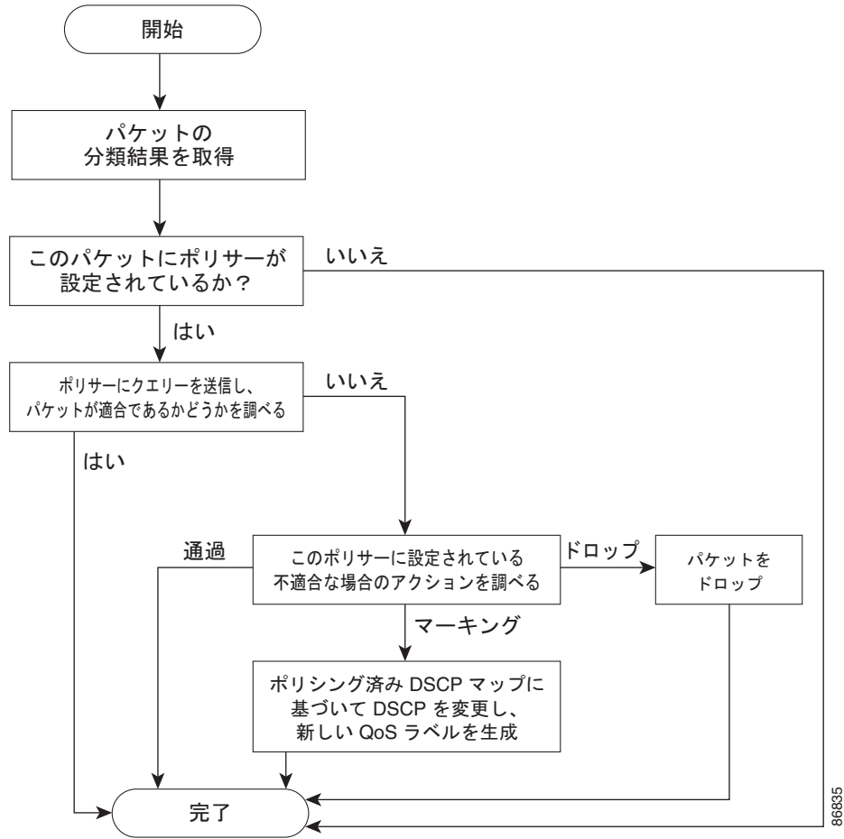
図 33-3 分類フローチャート
