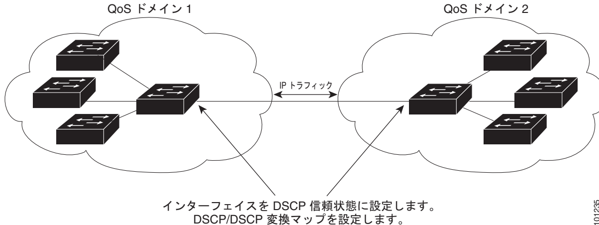
図 33-13 別の QoS ドメインとの境界ポートの DSCP 信頼状態
