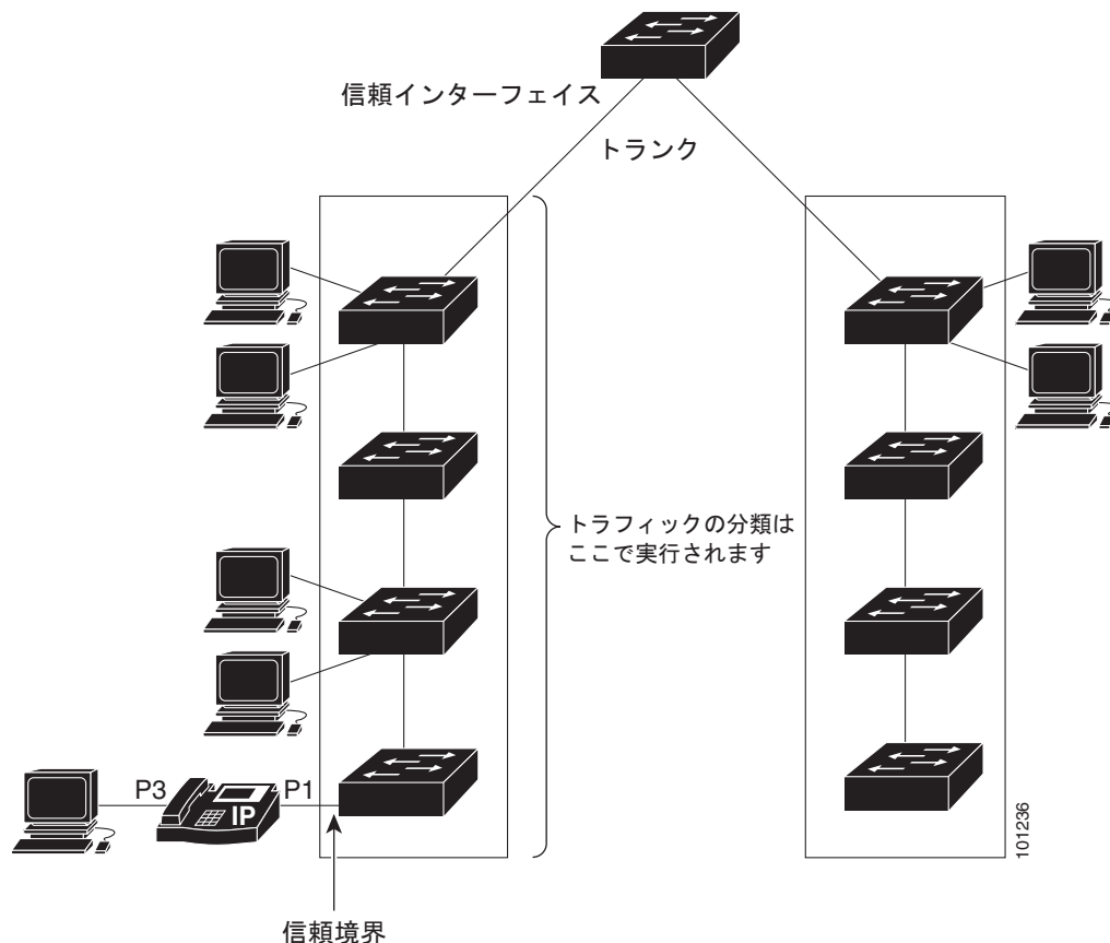
図 33-12 QoS ドメイン内のポートの信頼状態
