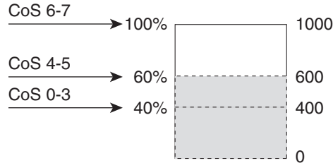
図 33-7 WTD およびキューの動作
