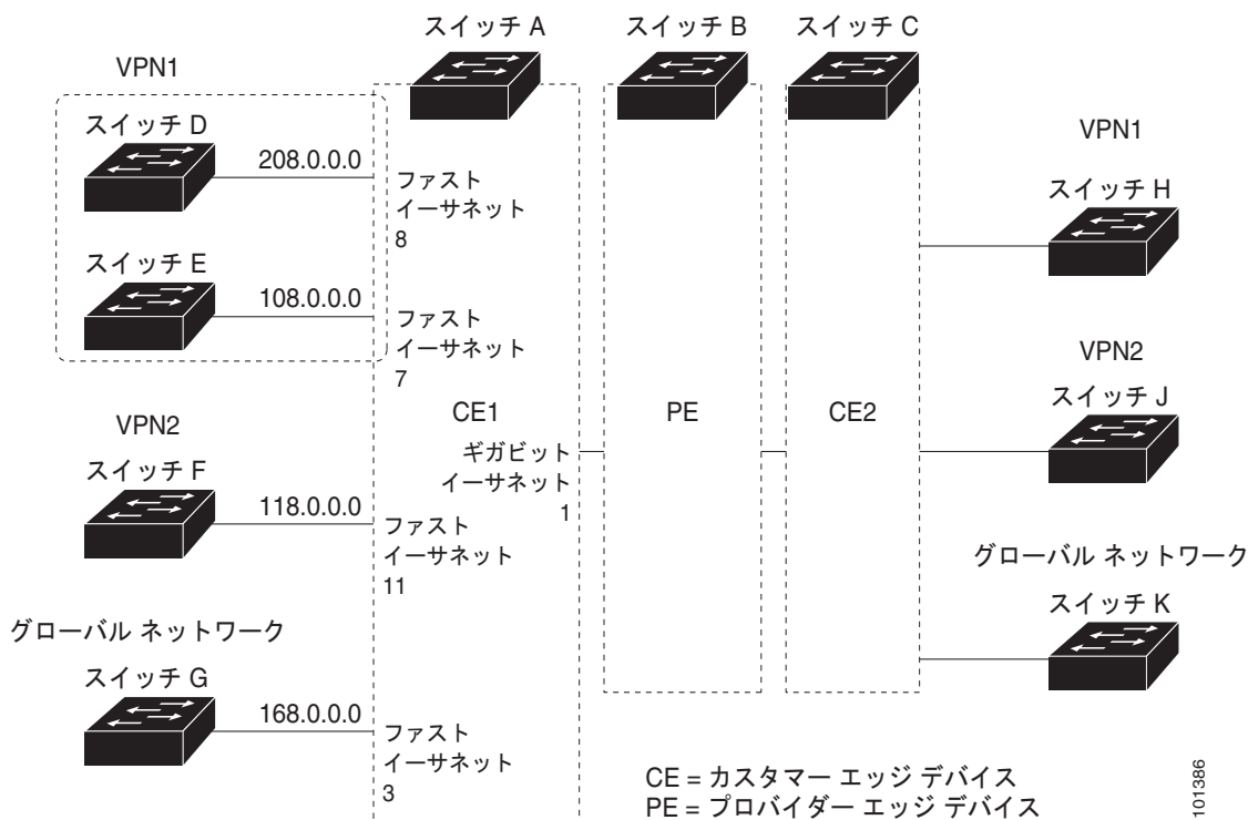
図 38-7 マルチ VRF CE の設定例
