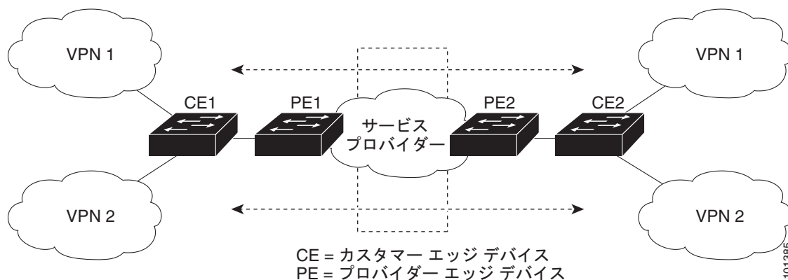
図 38-6 複数の仮想 CE として機能する Catalyst 3750 スイッチ
