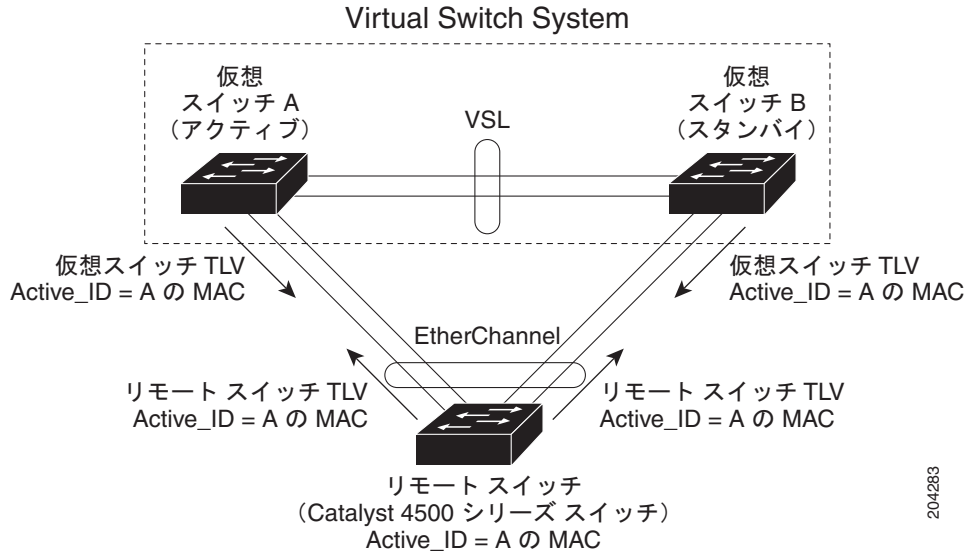
図 22-2 VSS のデュアルアクティブ シナリオでの拡張 PAgP
