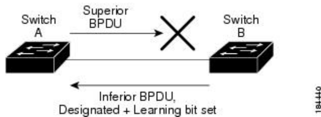
図 7: 単方向リンク障害の検出
