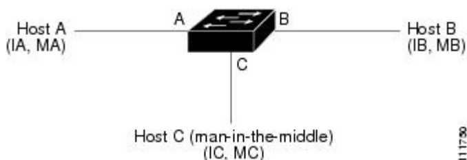
図 3: ARP キャッシュ ポイズニング
