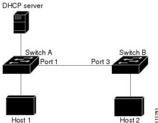
図 4: ダイナミック ARP インспекションのために有効にされた VLAN 上の ARP パケット検証
