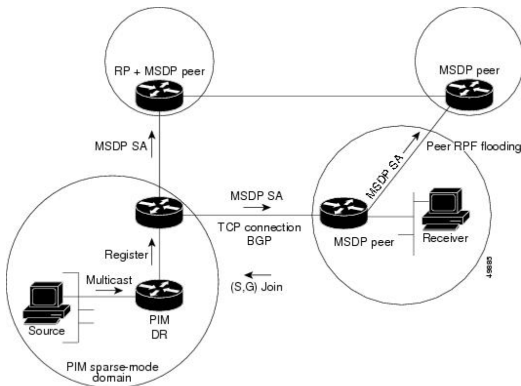
図 1: RP ピア間で動作する MSDP
