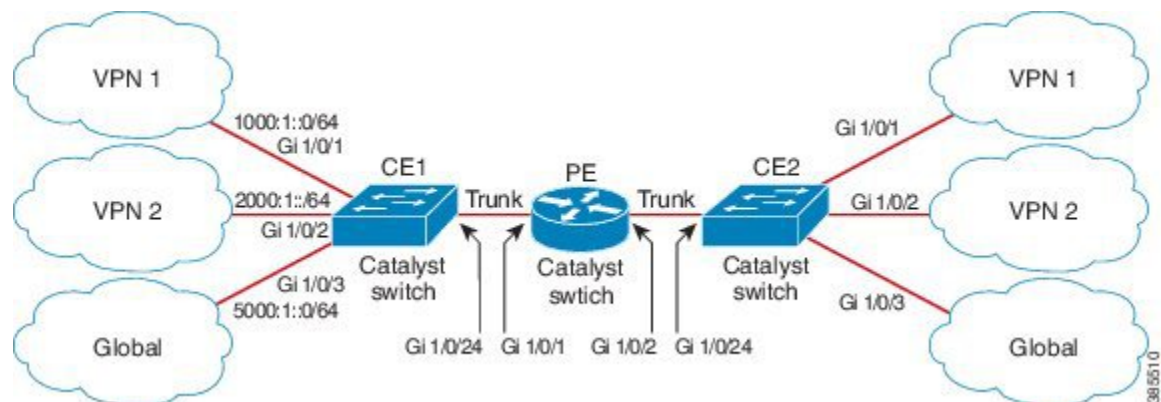
図 1: VRF-Lite の設定例
