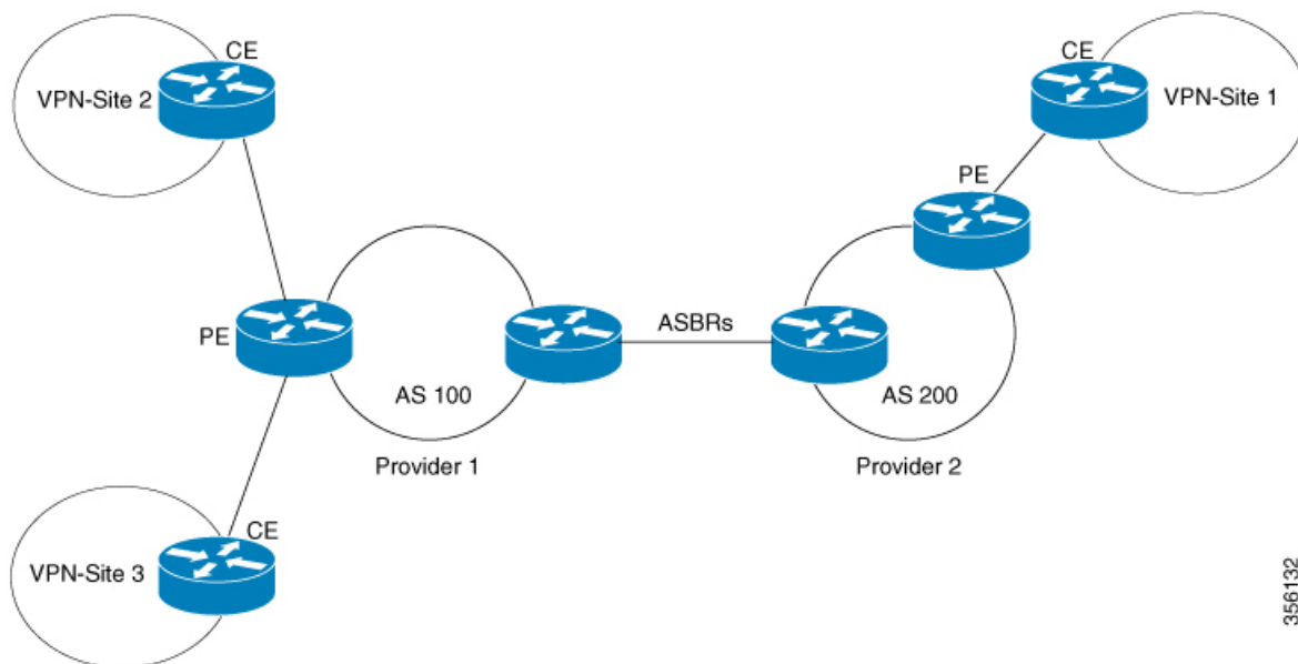
図 1: ネクストホップセルフ方式を使用した InterAS オプション B のトポロジ
