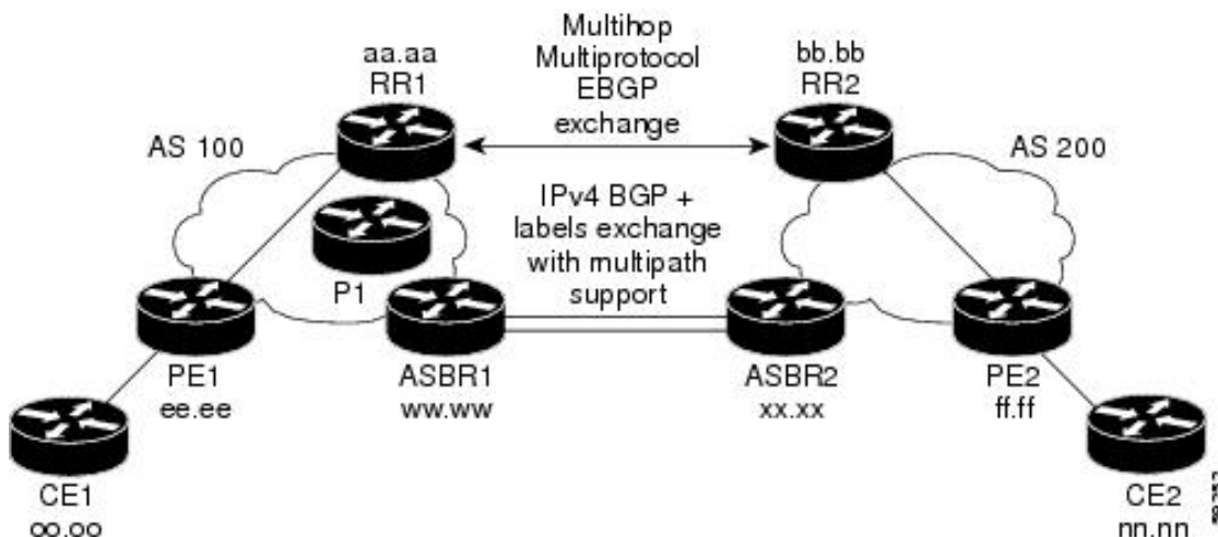
図 4: MPLS VPN サービスプロバイダー間での IPv4 ルートと MPLS ラベルの配布
