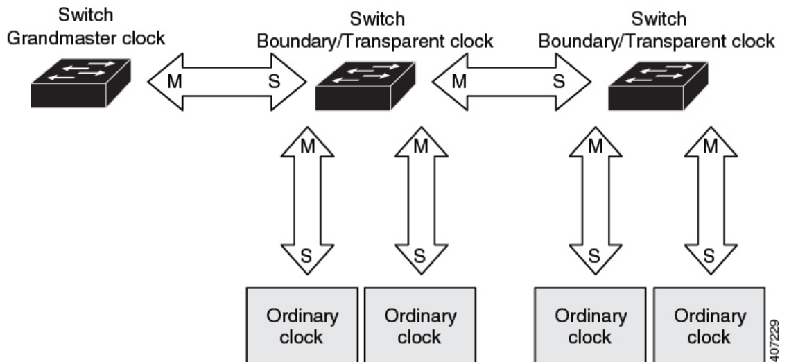
図 4: PTP クロック階層
