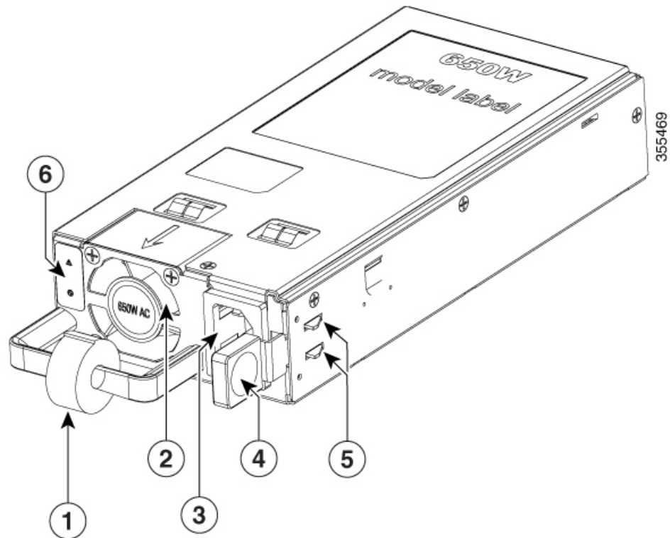
図 1: Cisco Catalyst 650W AC 入力電源モジュール
