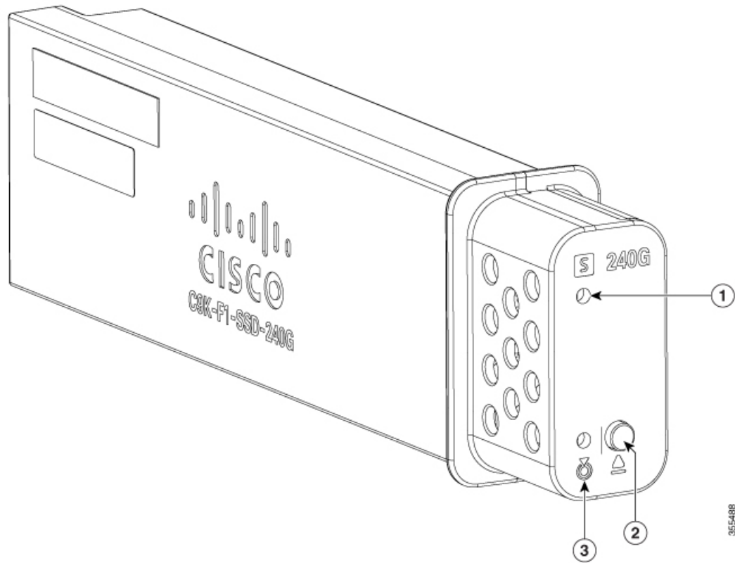
図 14: SATA SSD
