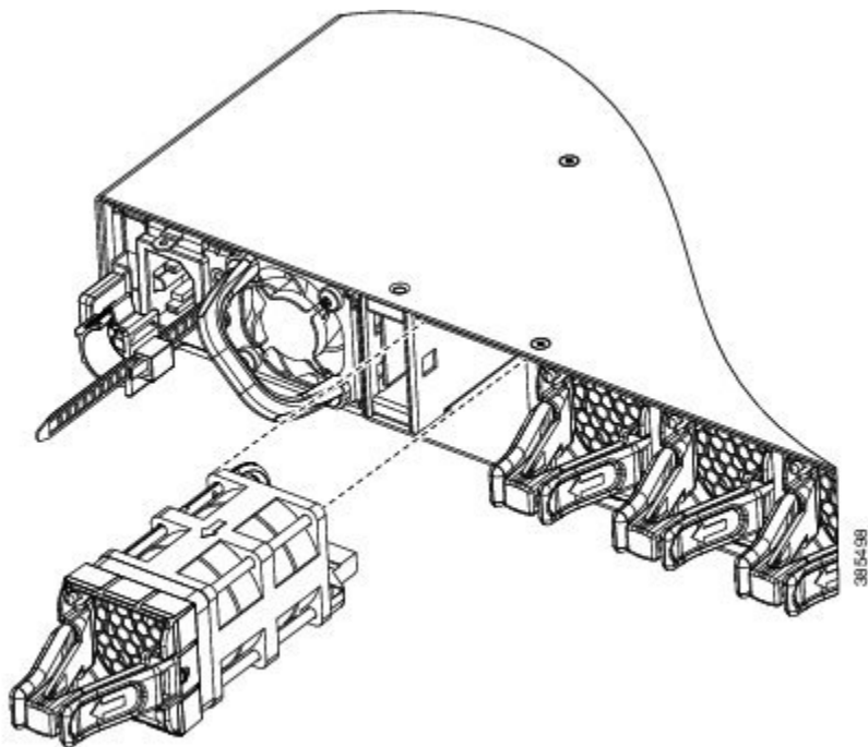
図 12: ファンモジュールの取り付け
