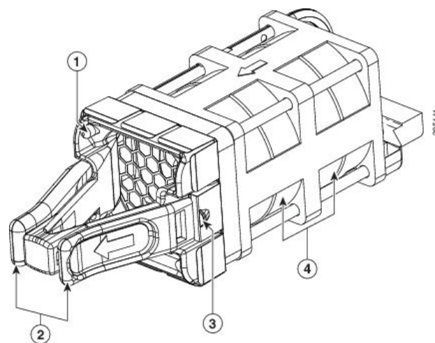
図 10: FAN-T4-R ファンモジュール
