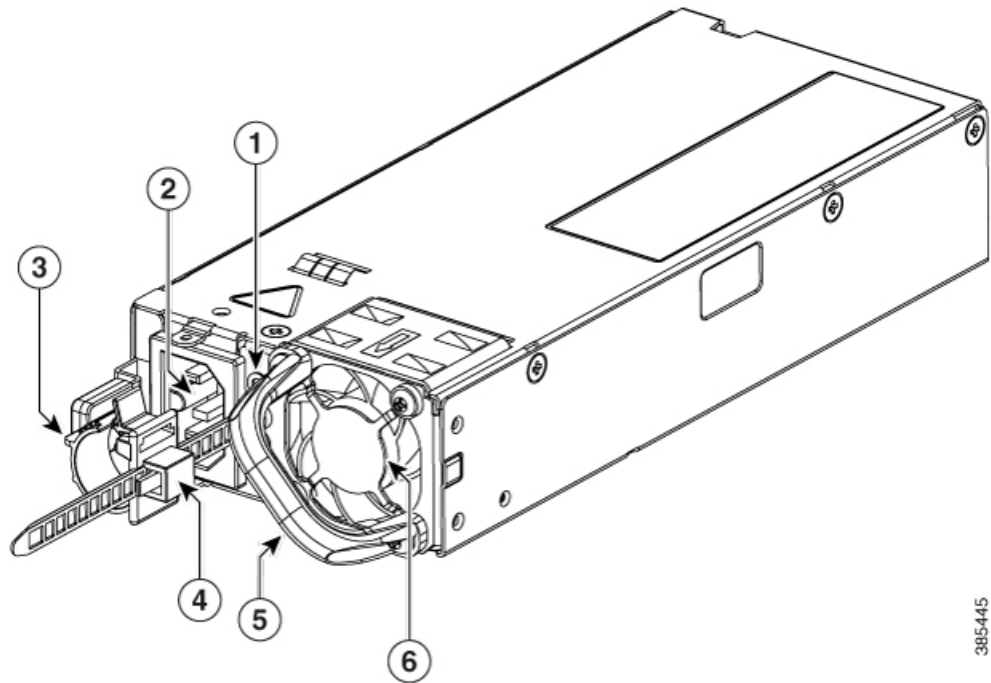
図 3: Cisco Catalyst 950W AC 入力電源モジュール
