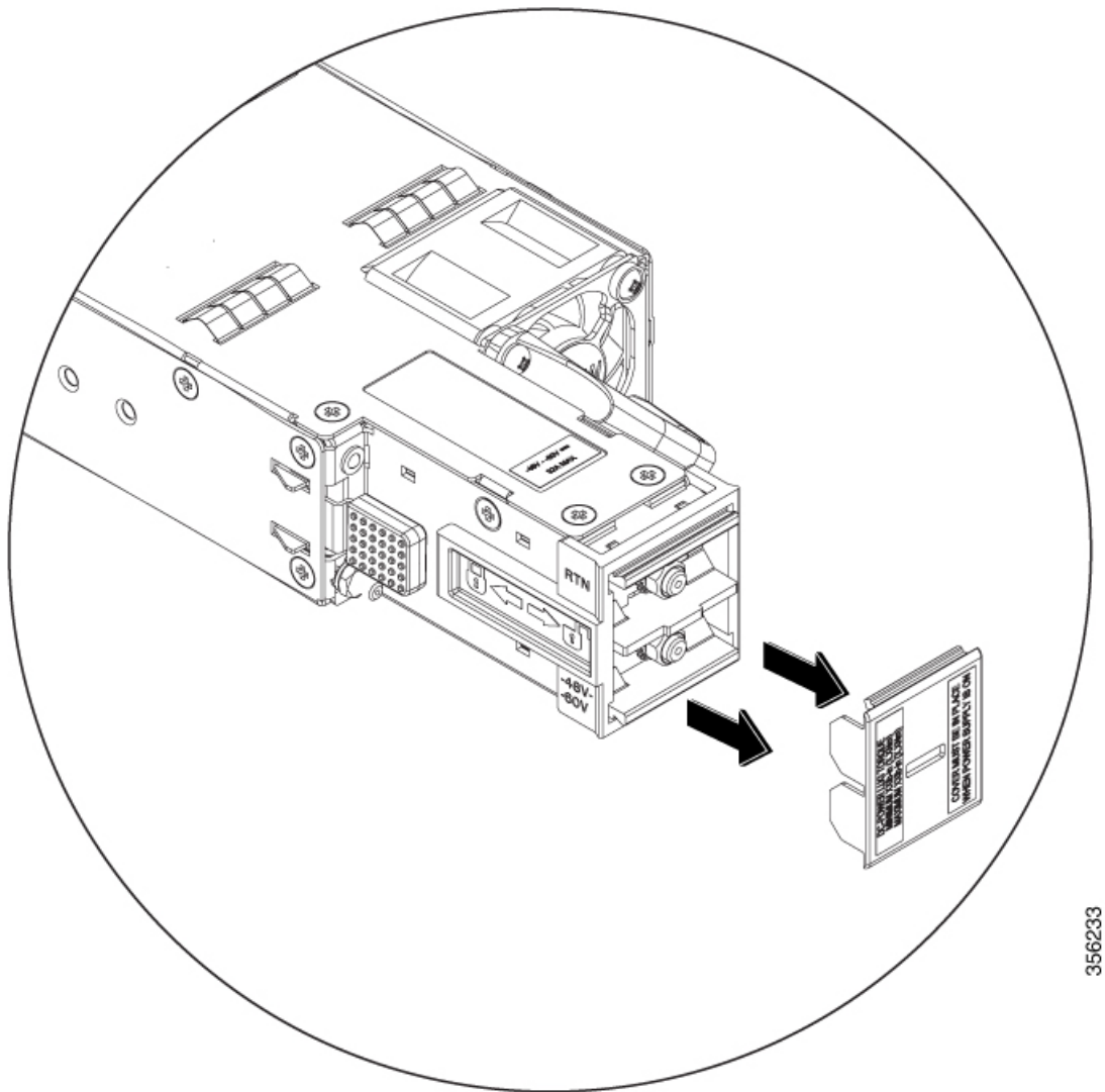
図 7: 保護カバーを取り外します。
