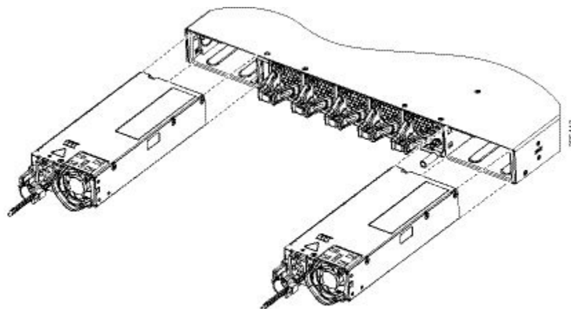
図 6: 電源装置の取り付け
