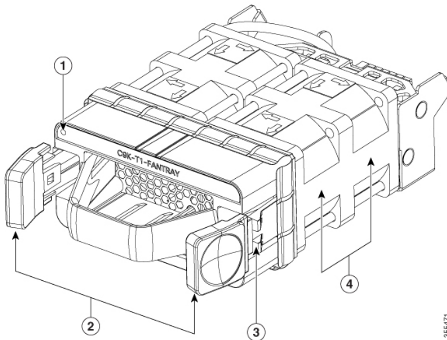
図 11:デュアルスタックファン付きファントレイユニット
