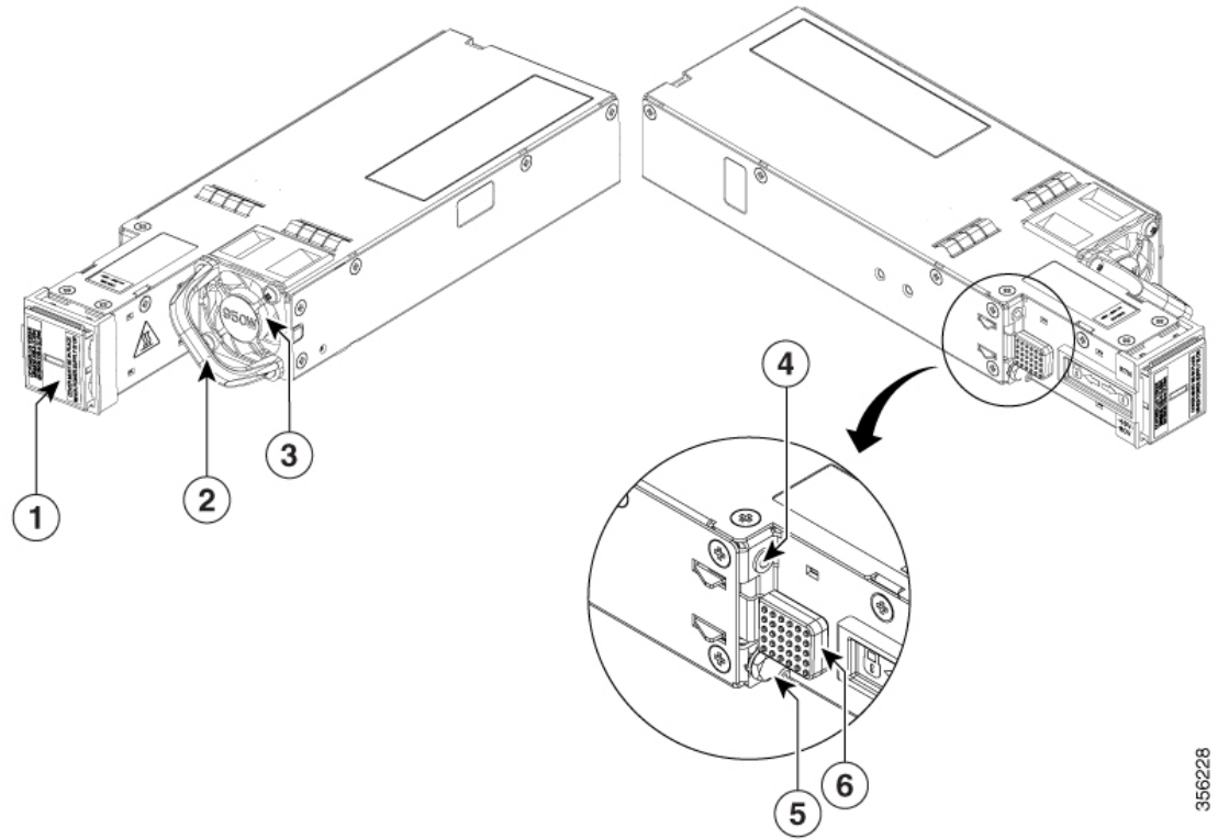
図 4: Cisco Catalyst 950W DC 入力電源モジュール
