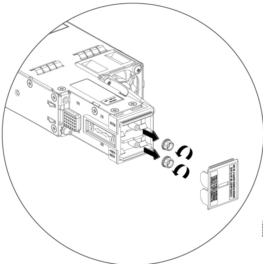
図 8: 端子ボックスのナットの取り外し
