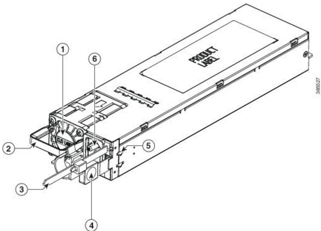
図 2 : Cisco Catalyst 1600W AC 入力電源モジュール
