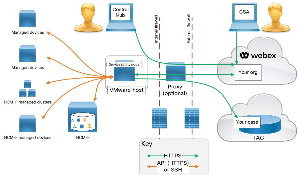
図 3: Expressway でのサービス コネクタを使用した展開
