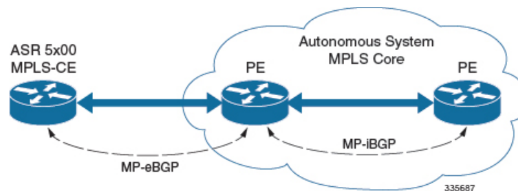
図 1: ASR 5500VPC-SI MPLS-CE から PE
