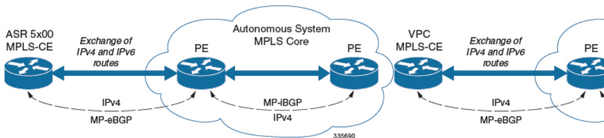
図 4: VPNv6 に対する IPv6-RD サポート
