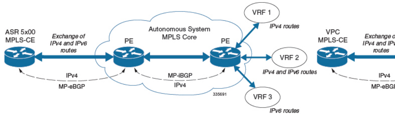
図 5: VPNv6 の設定例
