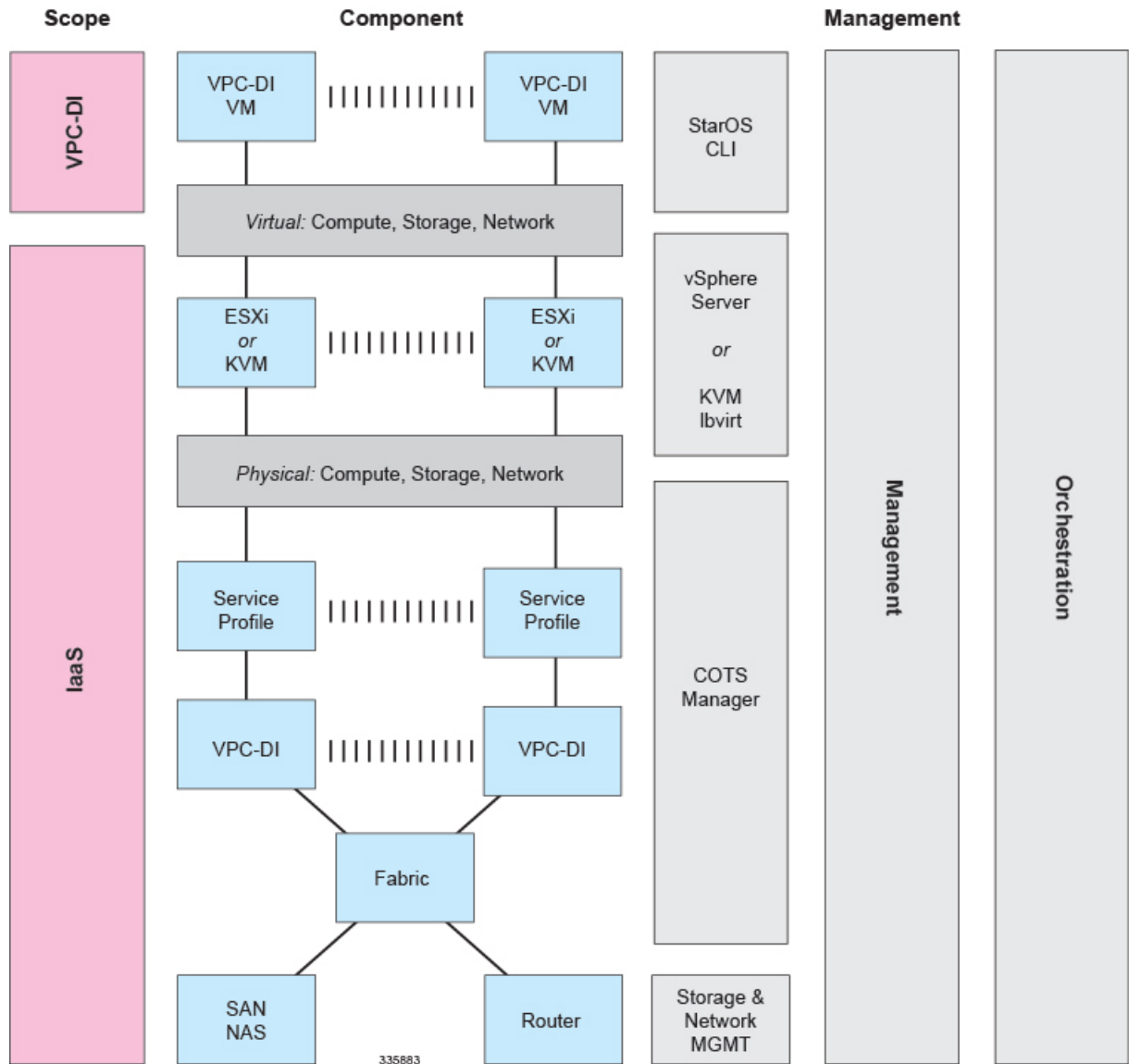
図 1: VPC-DI の範囲
