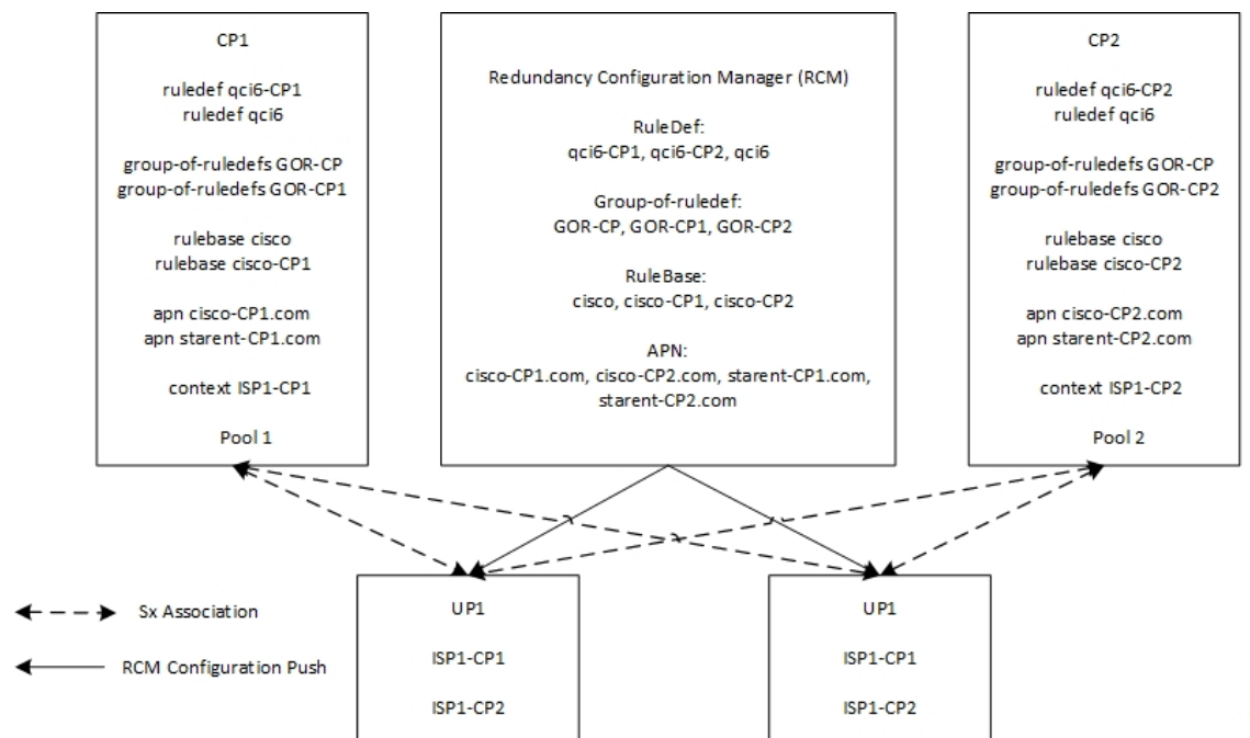
図 1: 2つの UP と通信する2つの CP の RCM 設定例
