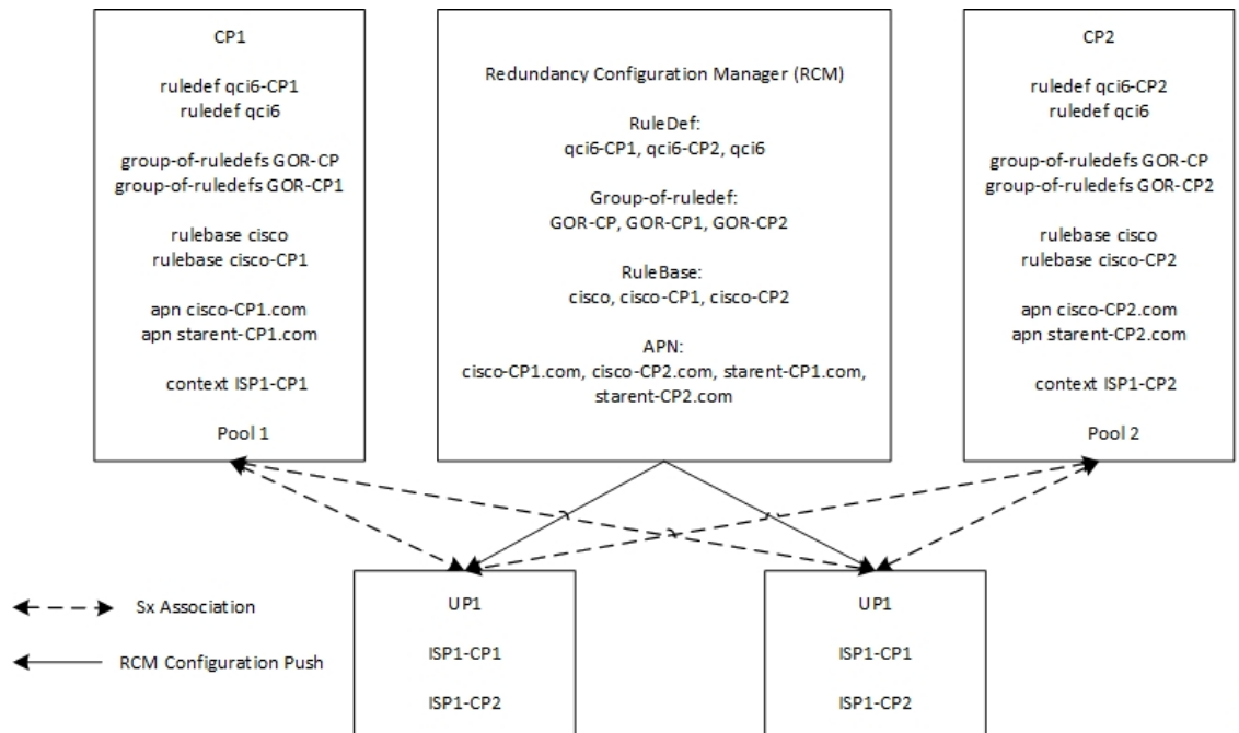
図 1: 2つの UP と通信する2つの CP の RCM 設定例
