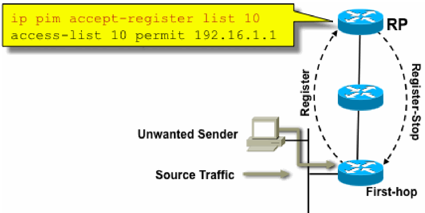
그림 17: PIM-SM 소스 제어
