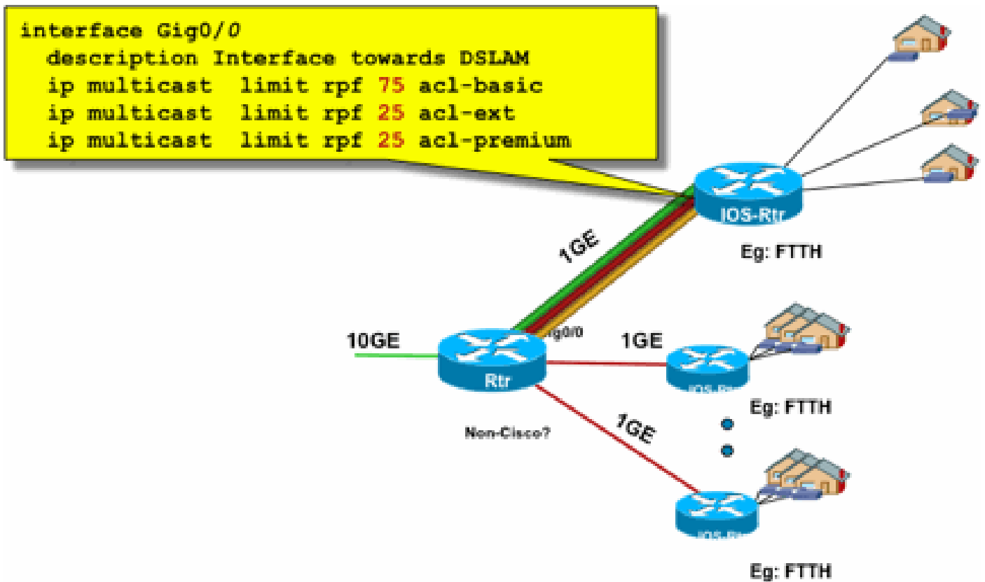
그림 22: 인터페이스별 경로 제한 사용, Input Admission Control
