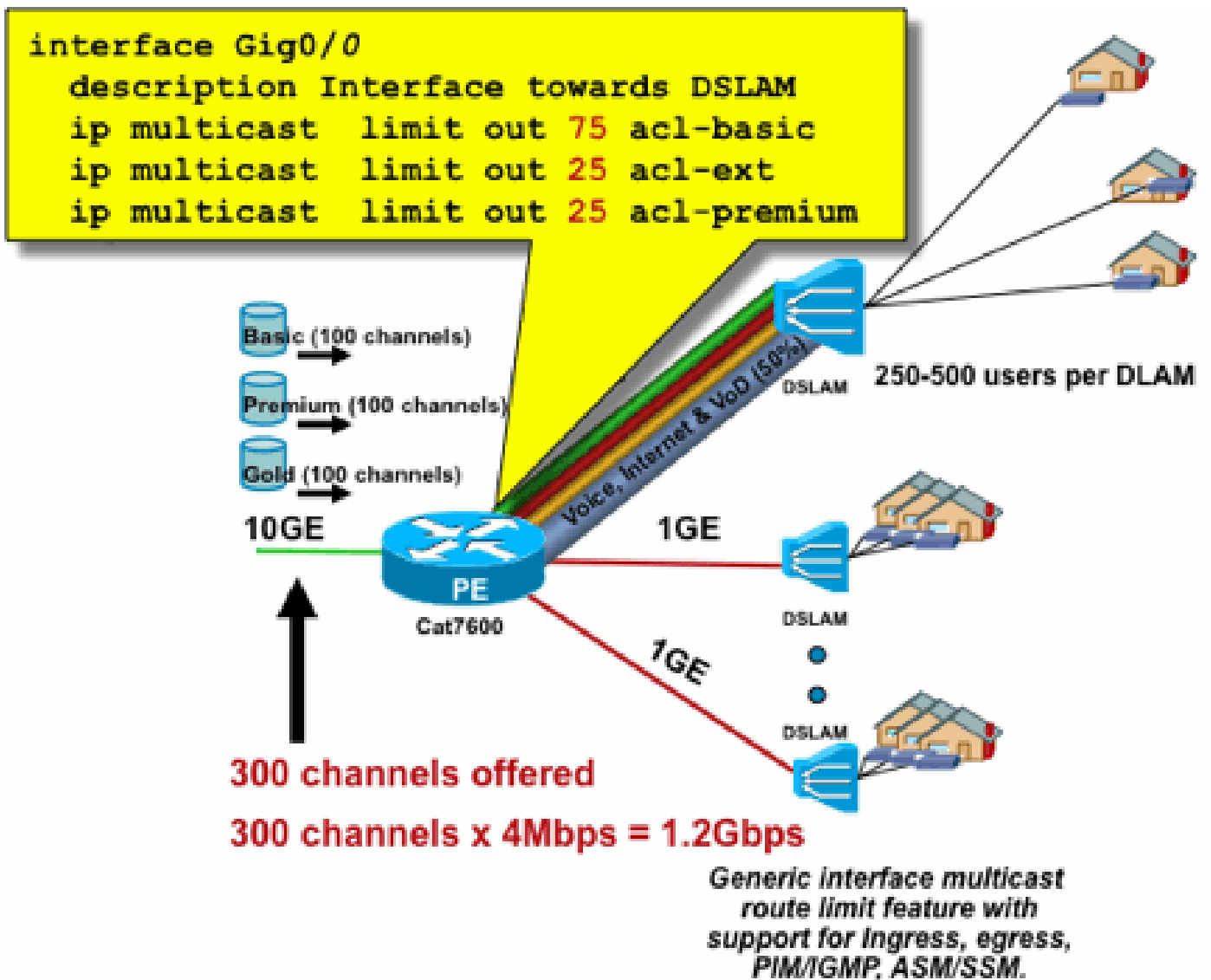
예 2 - Agg-DSLAM 링크의 Ingress Admission Control
