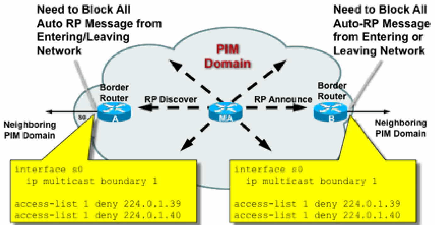
그림 10: 멀티캐스트 경계 명령
