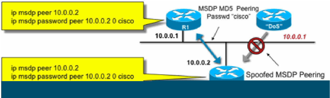
그림 15: MSDP MD5 네이버 인증
