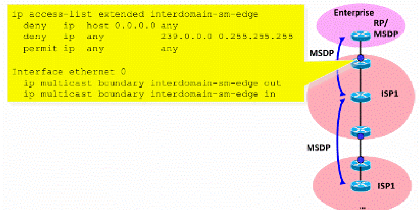
그림 13: 도메인 간(*,G) 필터
