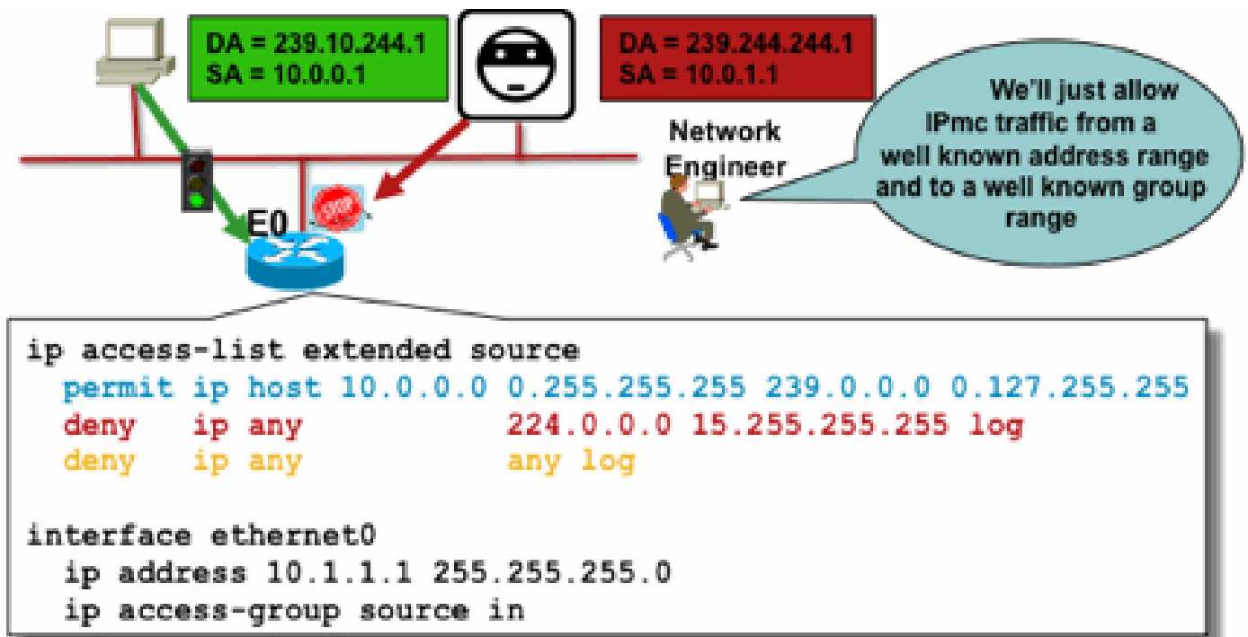
그림 16: 제어 소스
