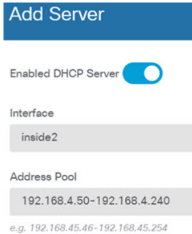
그림 4: DHCP 서버
