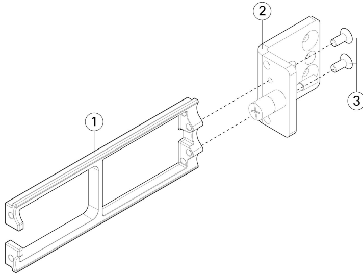
그림 2: 슬라이드 레일 잠금 브래킷에 케이블 관리 나사 설치
