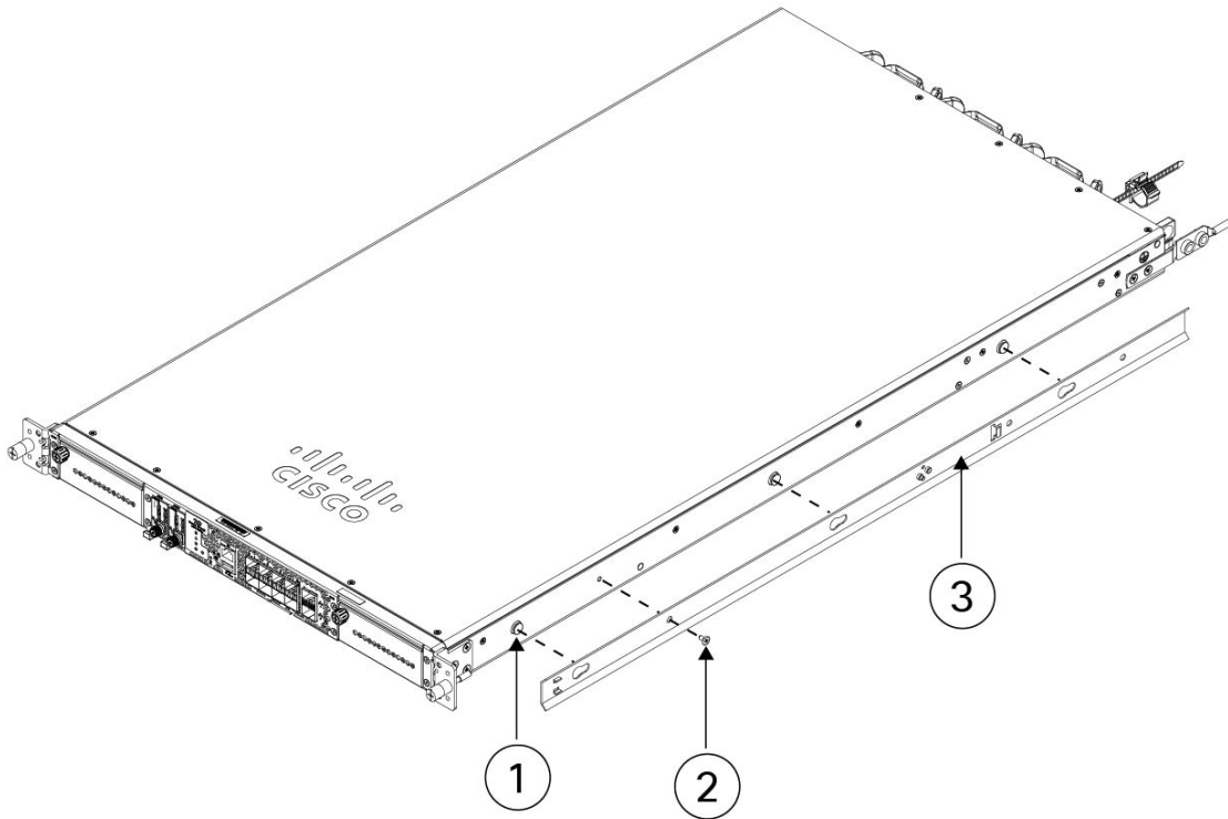
그림 3: 새시의 페그와 안쪽 레일 일렬로 맞추기
